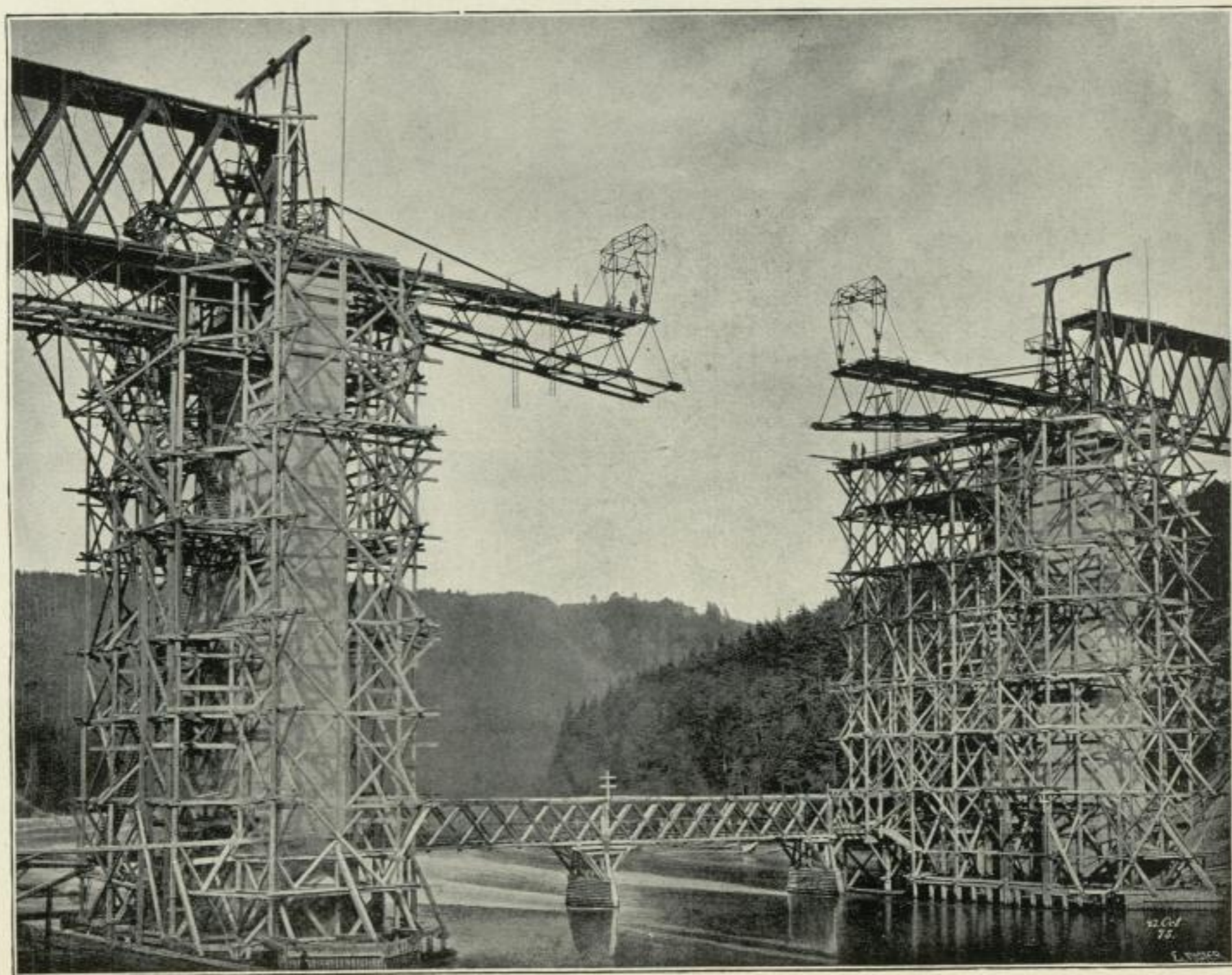
Eisenbahnbrücke über den Inn bei Königswart. Erbaut 1875/76.
