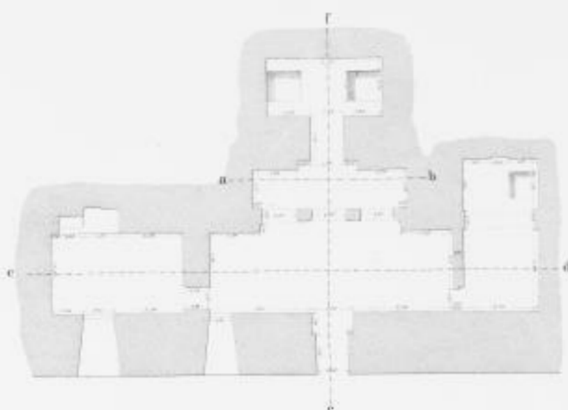
Grundriss.
