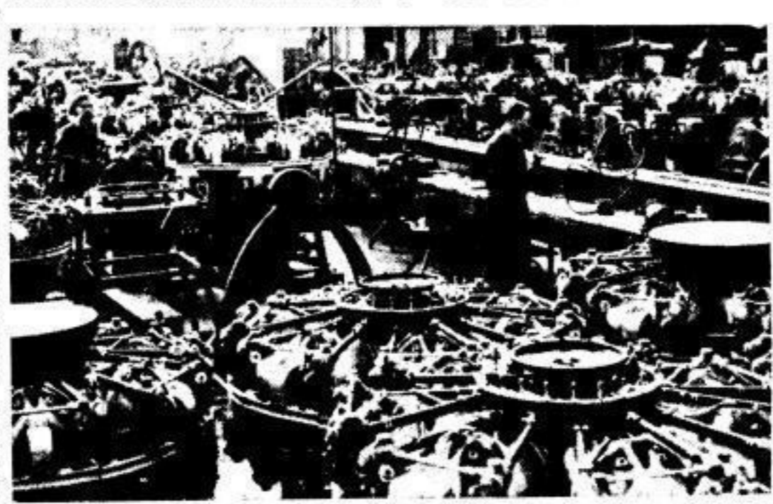
Flugmotoren entstehen in Großreihenfertigung. Einige tausend Teile birgt der BMW-Doppelsternmotor, das stählerne Herz der schnellsten deutschen Jagd- und Kampfflugzeuge, ein wahres Wunderwerk der Technik.
