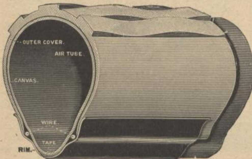
Dunlop-Reifen mit Welchs Antislippingmantel.
