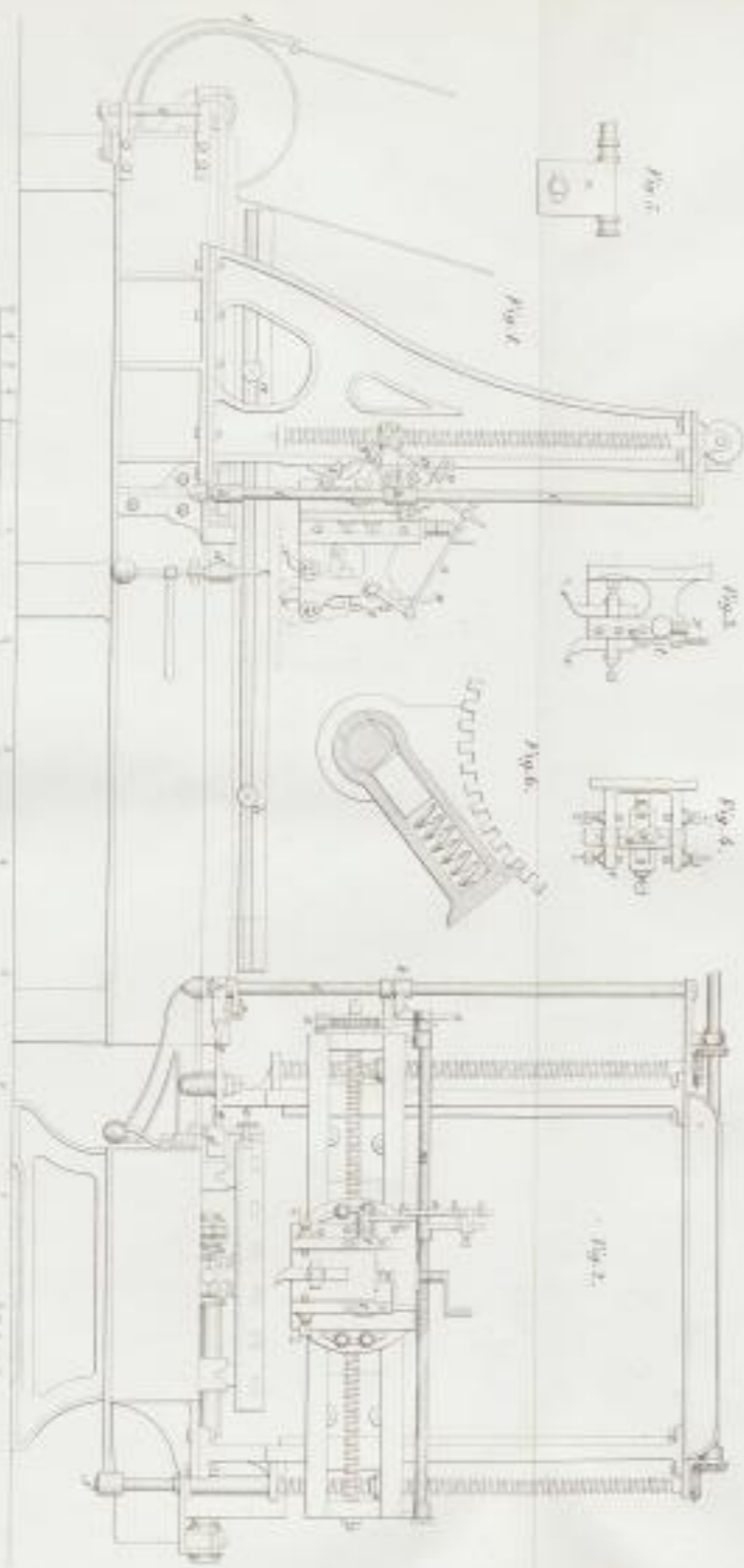
Metal-Handmaschine zum Vor- und Rückschnitt.
