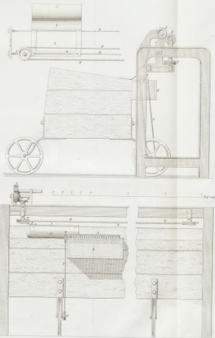
Mulemaschine für Baumwolle.
