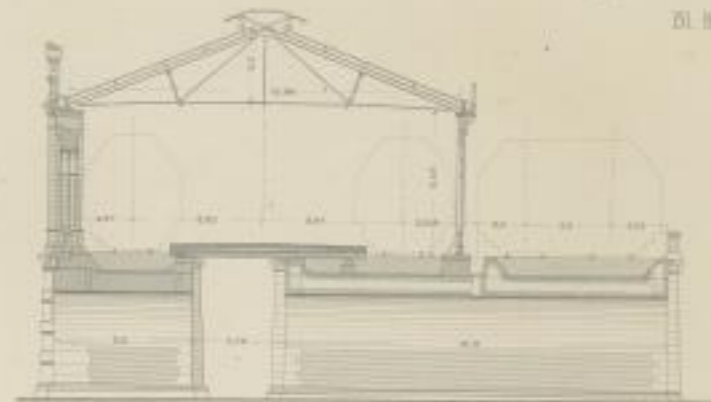
Schnitt durch die Halle
