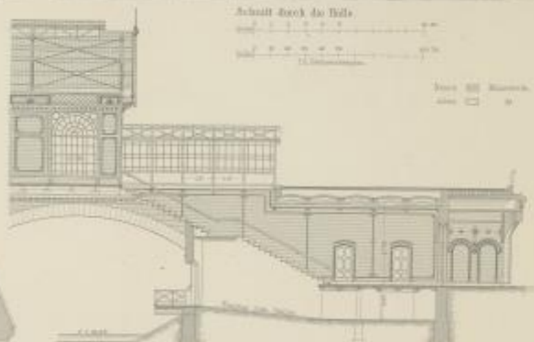
Schnitt cd
