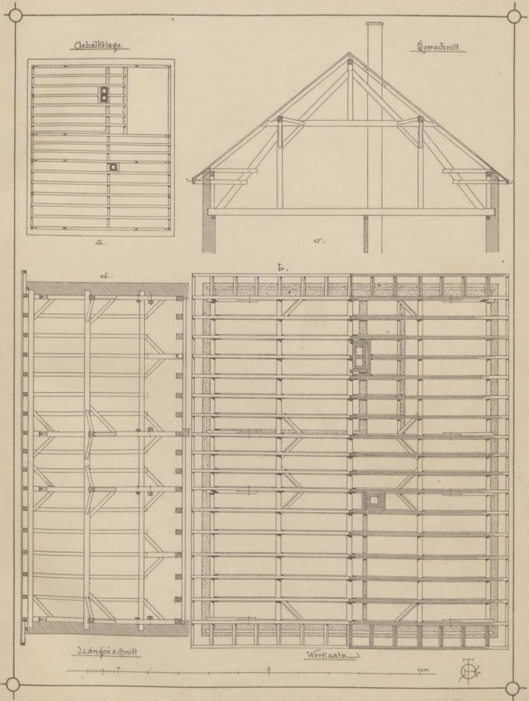
Werksatz eines stehenden Dachstuhles.
