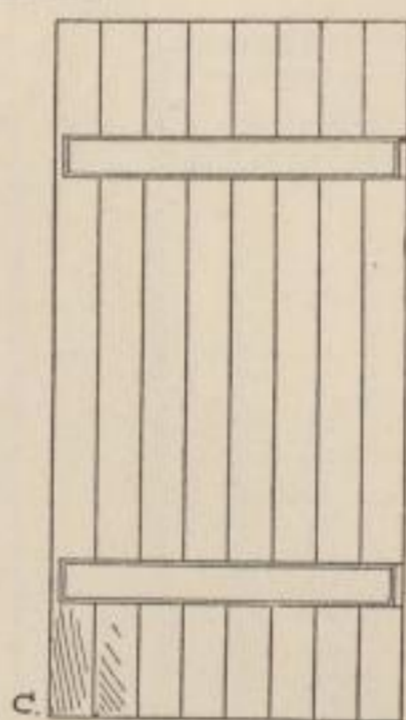
Stumpfverleimte Thüre mit Einschiebleisten
