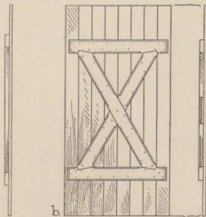
Riementhüre
