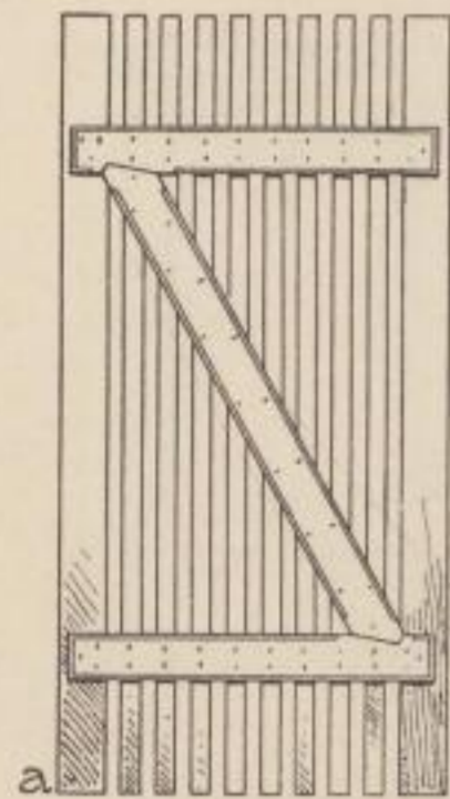
Lattenthüre
