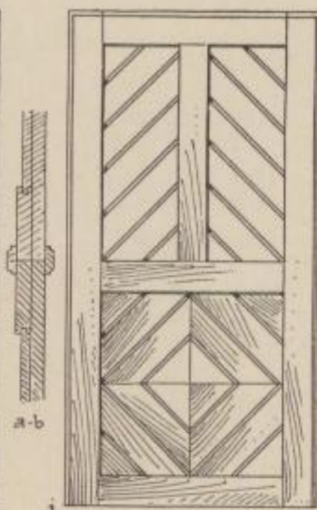
Verdoppelte Thüren für Keller, Waschkücher etc.
