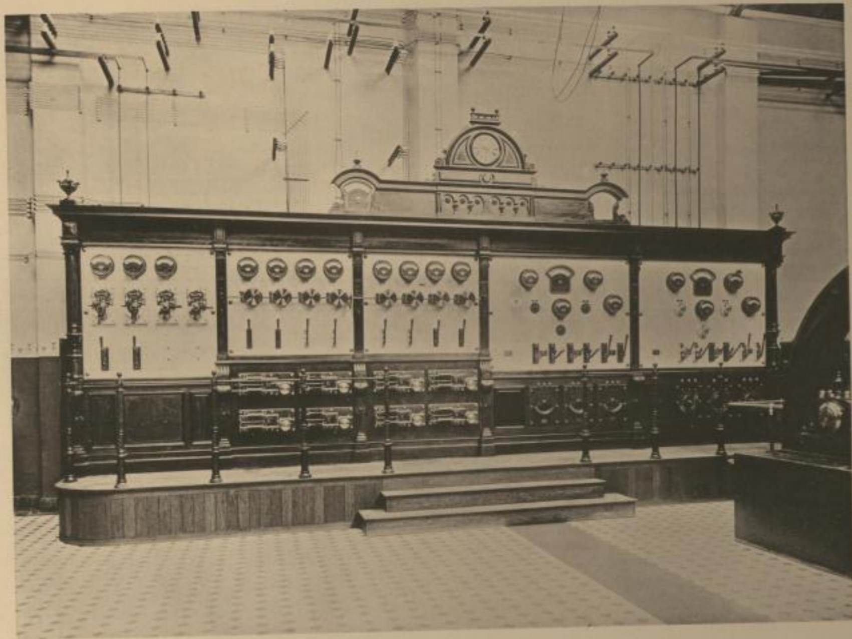
STRASSENBAHN HANNOVER IN HANNOVER SCHALTBRETT DER ACCUMULATOREN-LADESTATION VAHRENWALD
