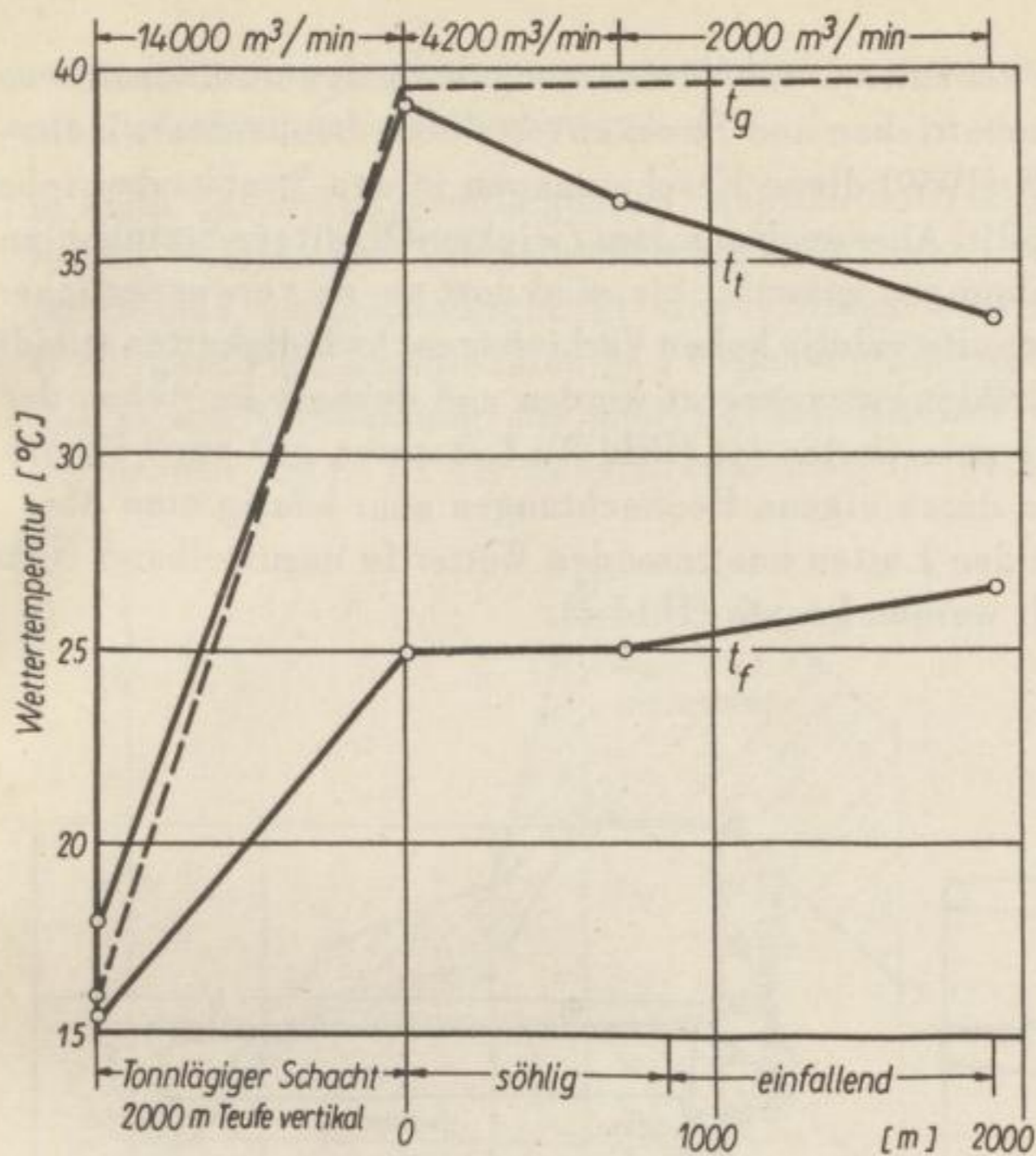
Bild 1. Mittlere Zustandsänderung der Wetter im einziehenden Wetterstrom einer tiefen Golderzgrube (BROMILOW 1954)
