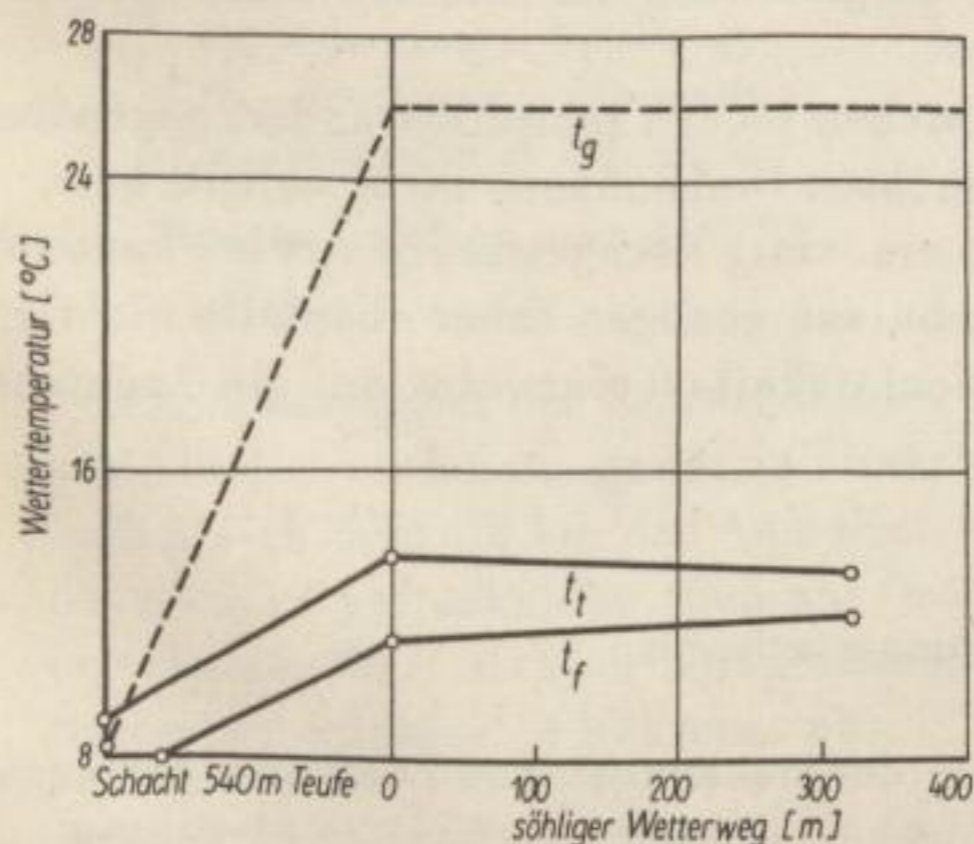
Bild 2. Mittlere Zustandsänderung der Wetter im einziehenden Wetterstrom einer Erzgrube (PIEHL 1964)
