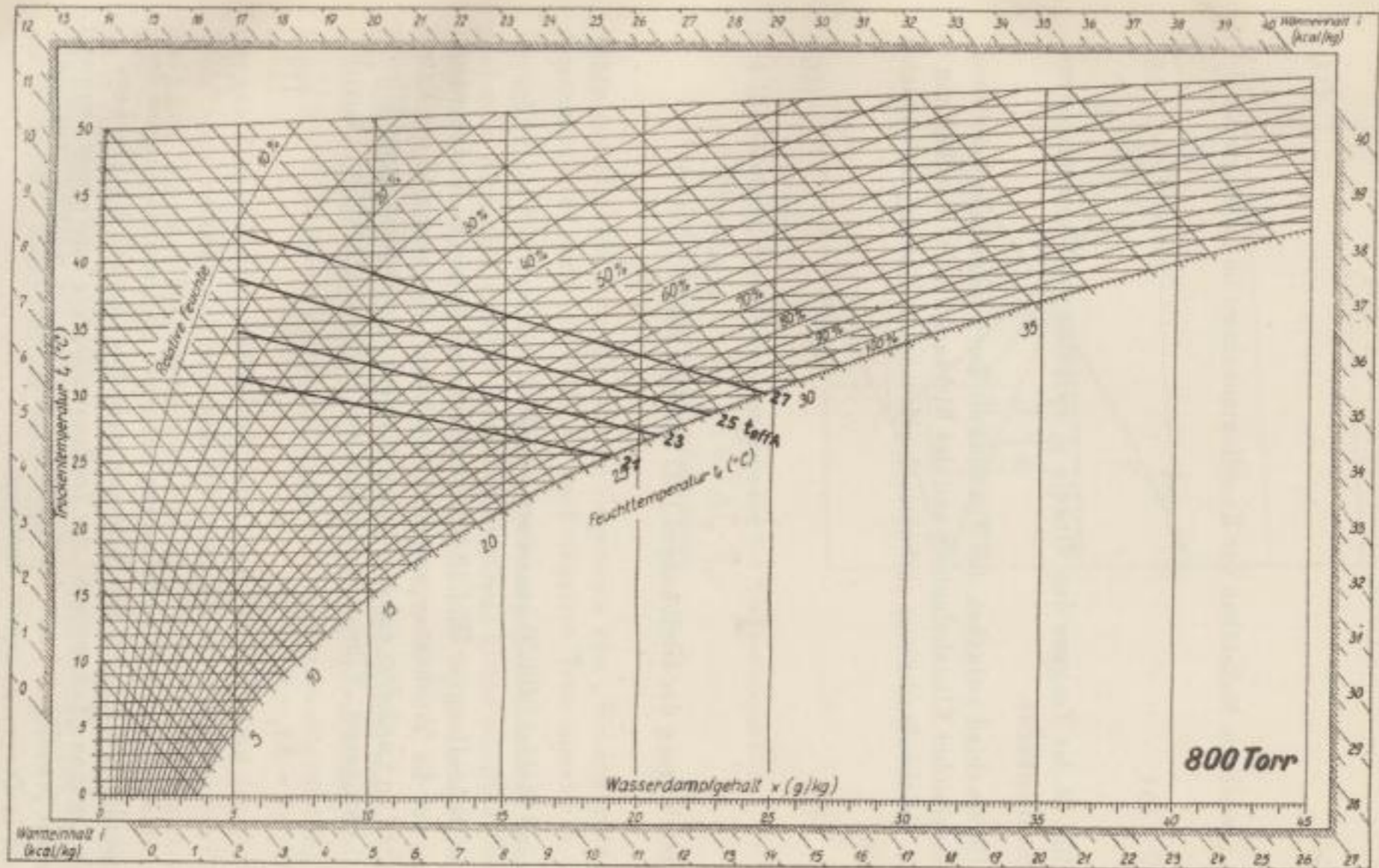
ix-Diagramm für Grubenwetter Tafel 2 zu Weuther, Faxl: Das ix-Diagramm und seine Anwendung bei grubenklimatischen Untersuchungen
