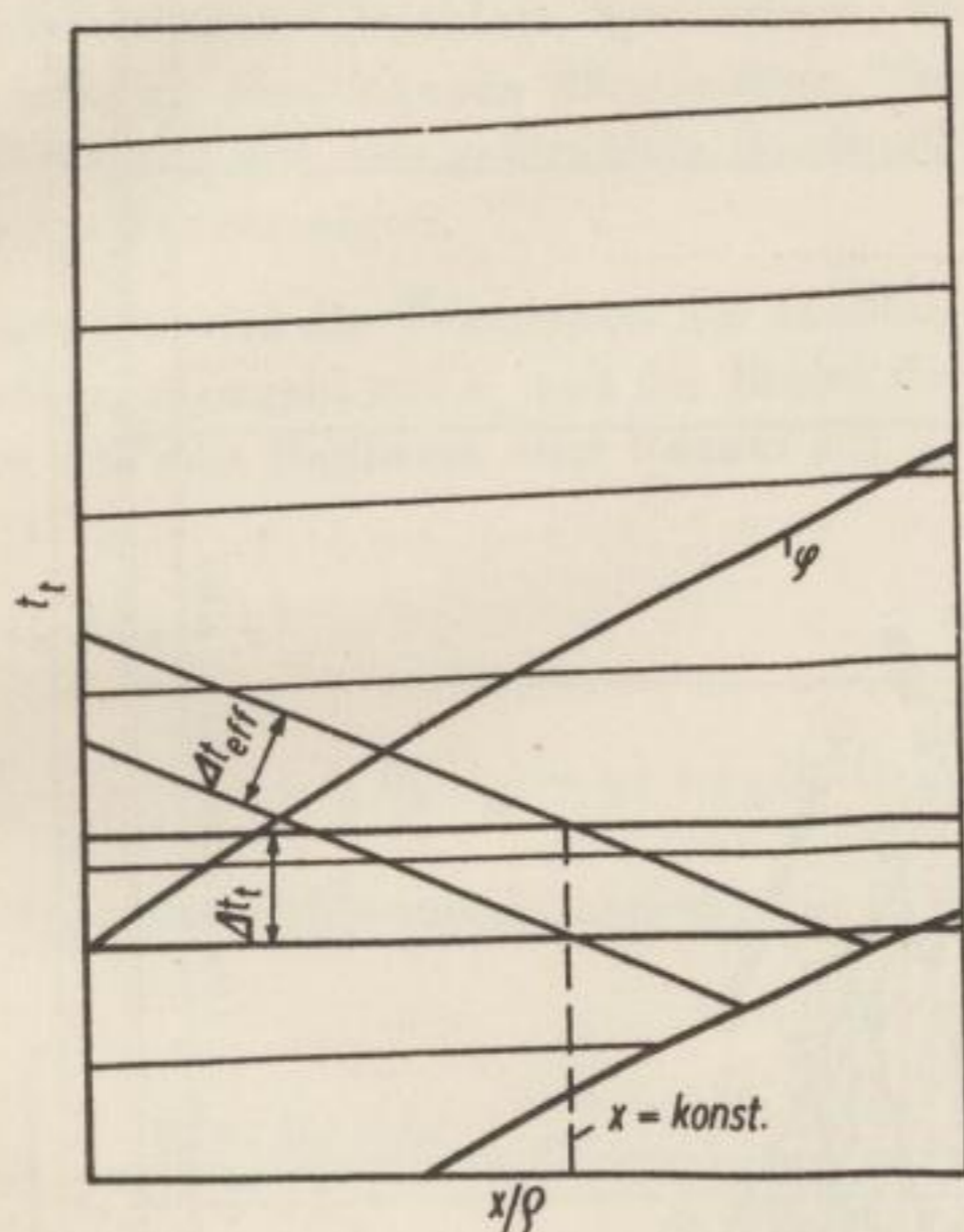
Bild 19. Beziehungen zwischen den Effektivtemperaturen und den Trockentemperaturen
