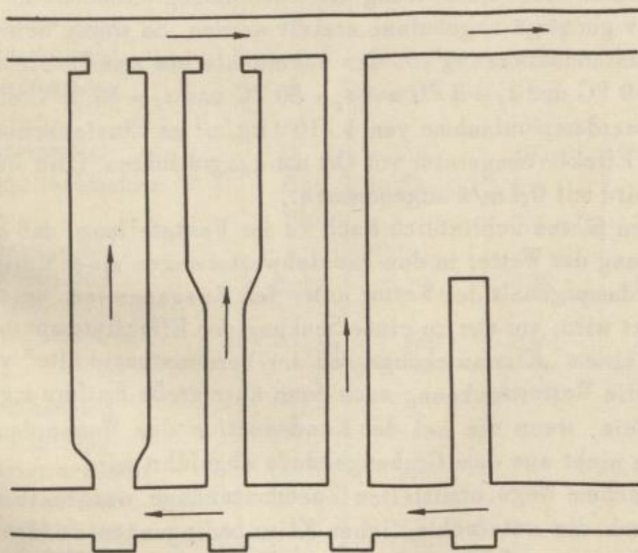
Bild 28. Schematische Darstellung bei verbesserter Wetterführung durch Änderung der Auffahrungsmethode der Abbaukammern im Kalibergbau
