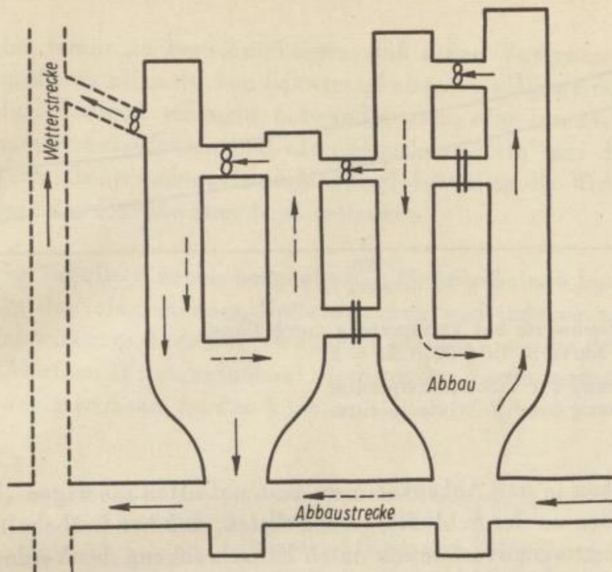
Bild 27. Schematische Darstellung der Wetterführung im Kalibergbau — Wetterstrom — — Wetterkreisläufe
