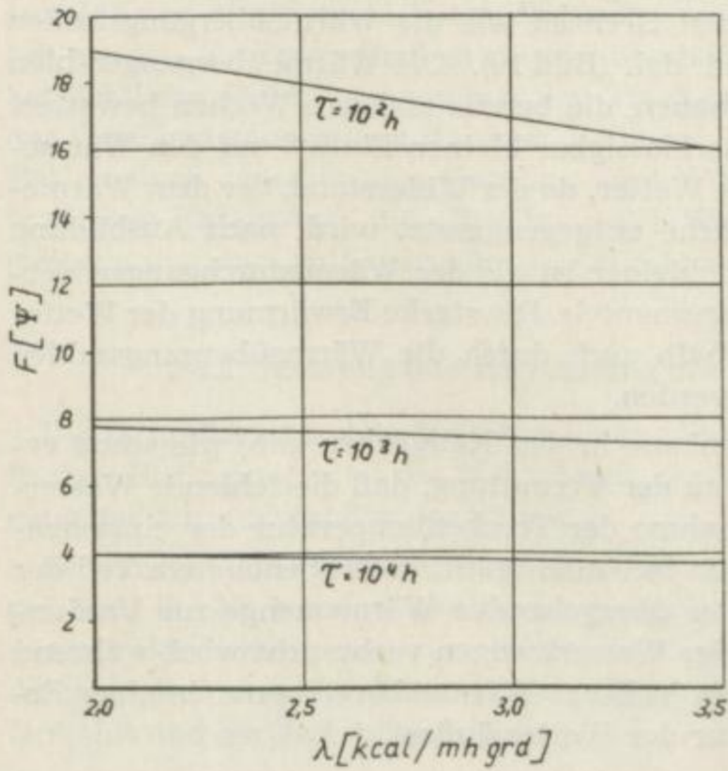
Bild 9 Abhängigkeit der Funktion des Altersbeiwertes von der Wärmeleitfähigkeit des Gesteins
