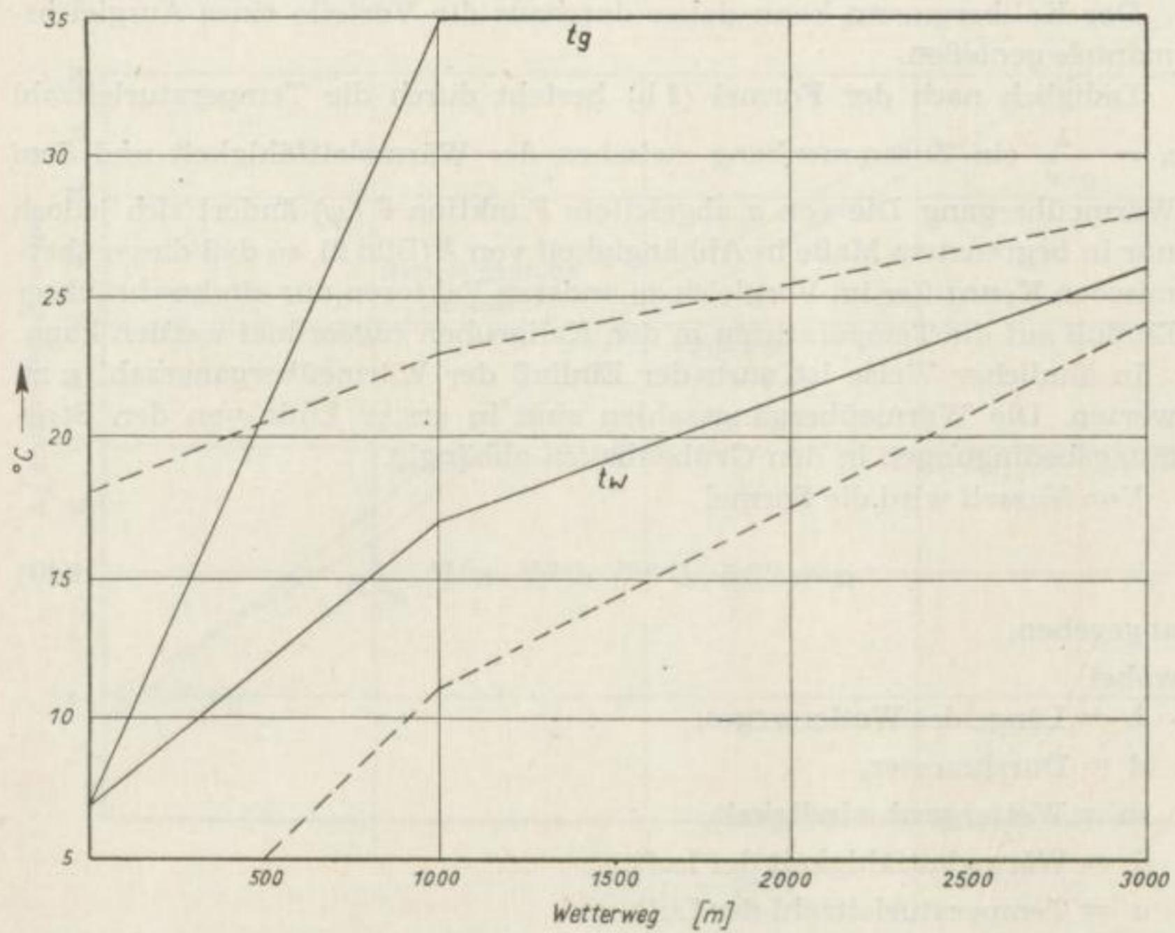
Bild 8. Wärmeausgleichsmantel
