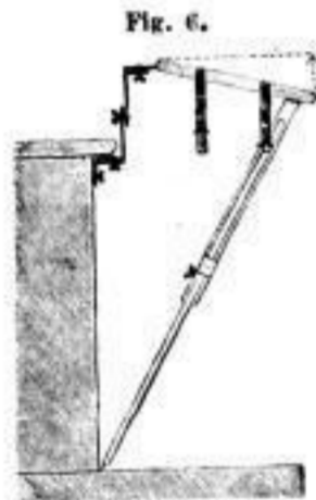
Höchste Stellung bei Benutzung als Stehpult.
