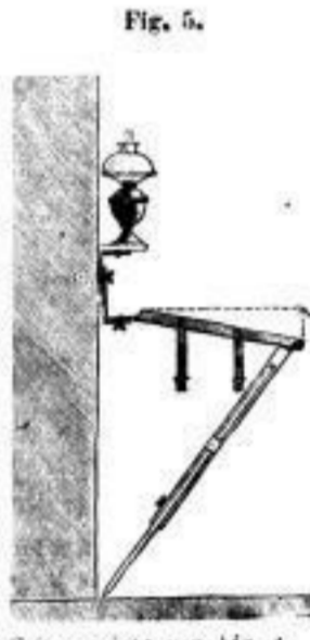
Seitenansicht von Fig. 4.
