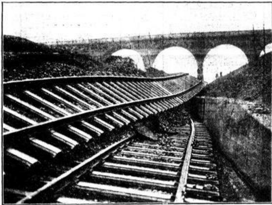
Der Dammrutsch bei Frankfurt a. Oder. Auf der Eisenbahnstrecke Berlin - Frankfurt stürzte der Bahndamm zwischen den Stationen Pilsom und Rosengarten in einer Länge von 150 Metern zusammen.
