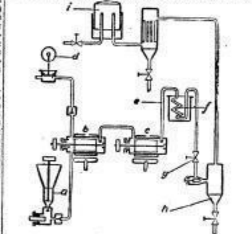
Verflüssigungsanlage.
