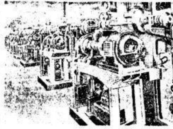
Multifunktionsmaschinen-Antrieb mit Haupt- und Hilfsmotoren nach AEG
