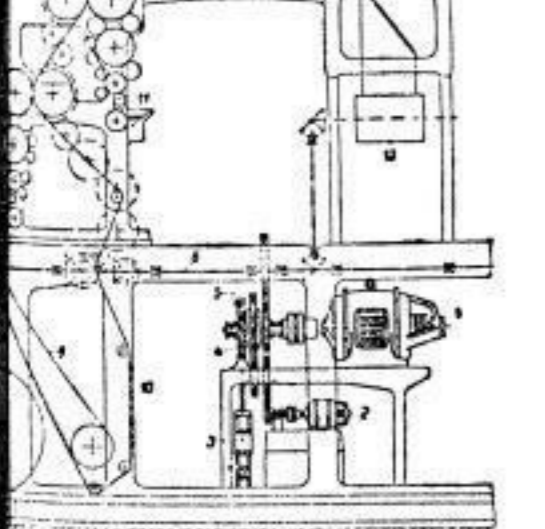
Antriebsanordnung einer Rotationsdruckmaschine nach AEG
