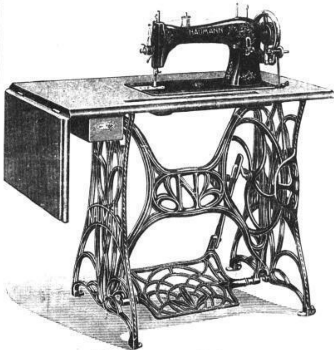
Naumann C 4 Zentralspulen-Fußnähmaschine für Tucharbeiten der Damen- und Herren- schneiderei sowie für leichtere Lederarbeiten. Das Gestell ist mit großem Schwungrad versehen. Die Maschine näht vor- und rückwärts. Durchgangsraum 30 x 15 cm. Größe der Tischplatte mit Klappe 130 x 48 cm.
