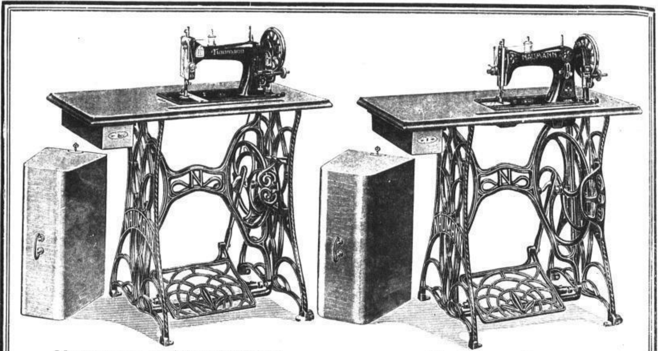
Naumann D 4 Zentralspulen - Fußnähmaschine für den Familiengebrauch, Damenschneiderei, Wäsche- und Trikotage-Näherei usw. Die Maschine näht vor- und rückwärts. Durchgangsraum: 22 x 13 cm. Größe der Tischplatte: 85 x 44 cm.
