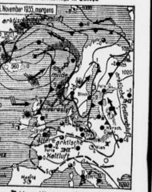
Die Wetterlage in Europa am 27. November 1935 morgens
