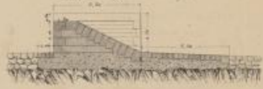
e. Fig. 8 Coupe sur xx Fig. 7
