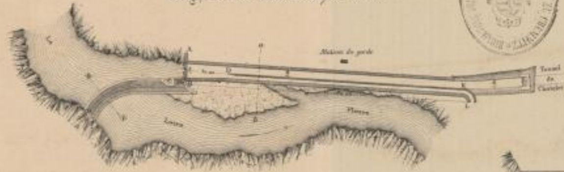
d. Fig. 7 Plan de détail de la prise d'eau
