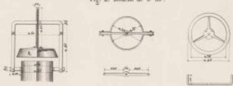
Fig. 2. Bouche de 0 m 30.
