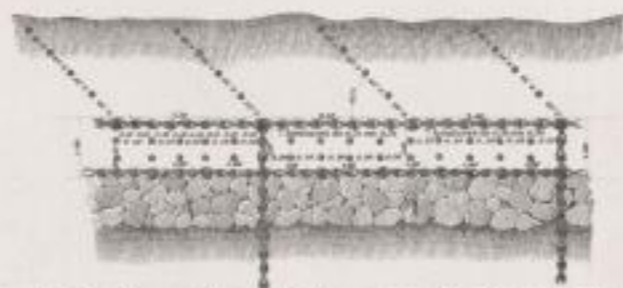
Fig. 4.— Plan du clayonnage longitudinal avec amorce des clayonnages transversaux et des lignes de butées.
