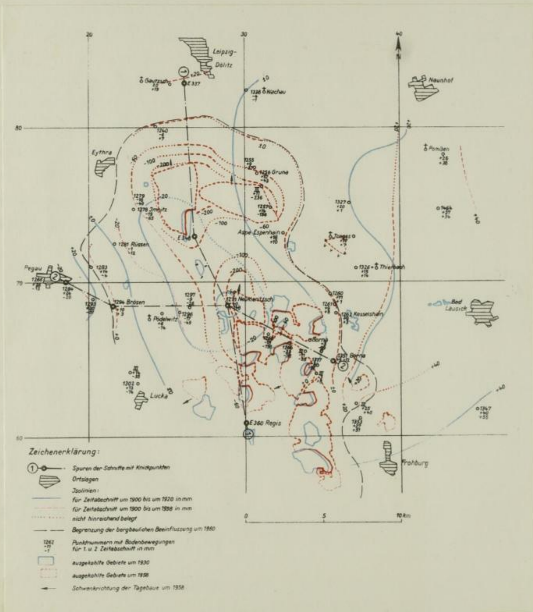
Bild 1 : Karte der vertikalen Bodenbewegungen im Vorfeld der Tagebaue im Braunkohlenrevier Borna
