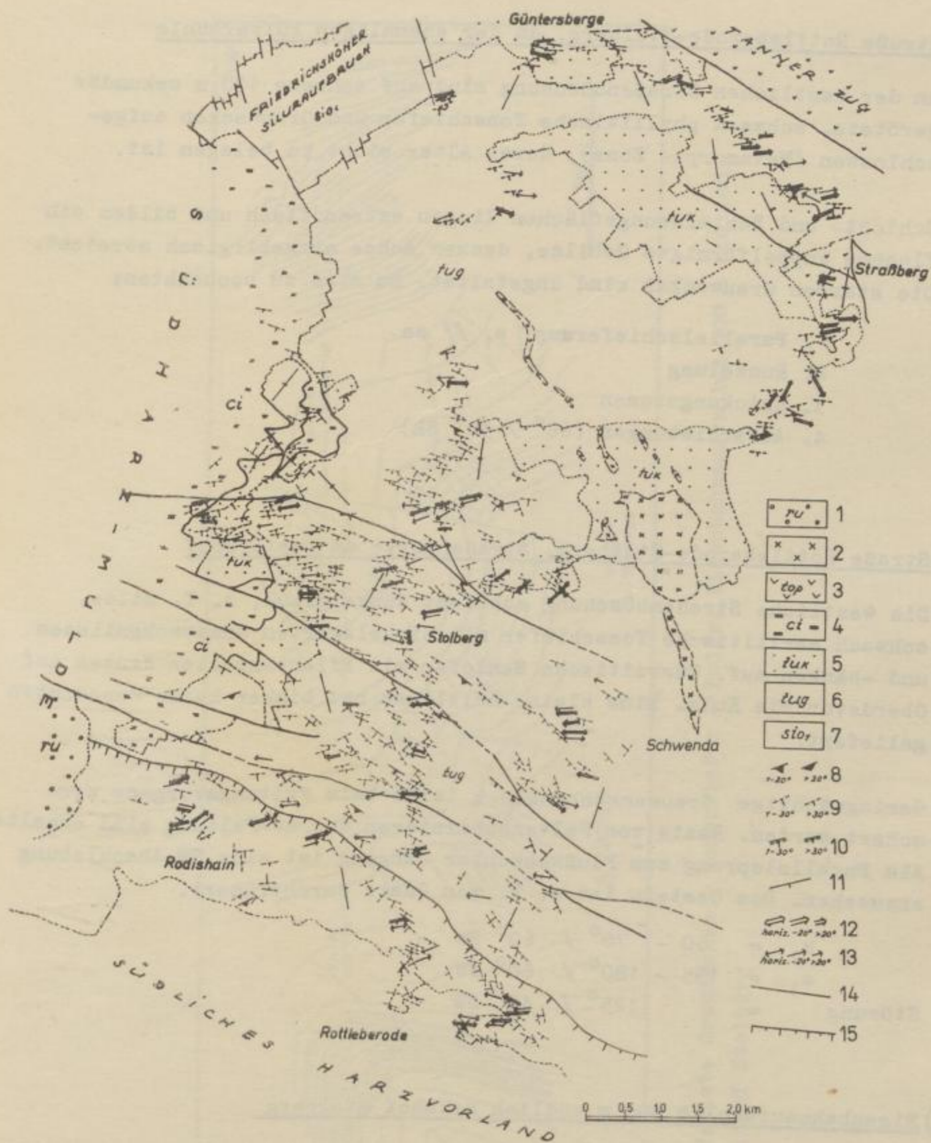
Abb. 5. Strukturkarte der westlichen Harzgeröder Faltenzone
