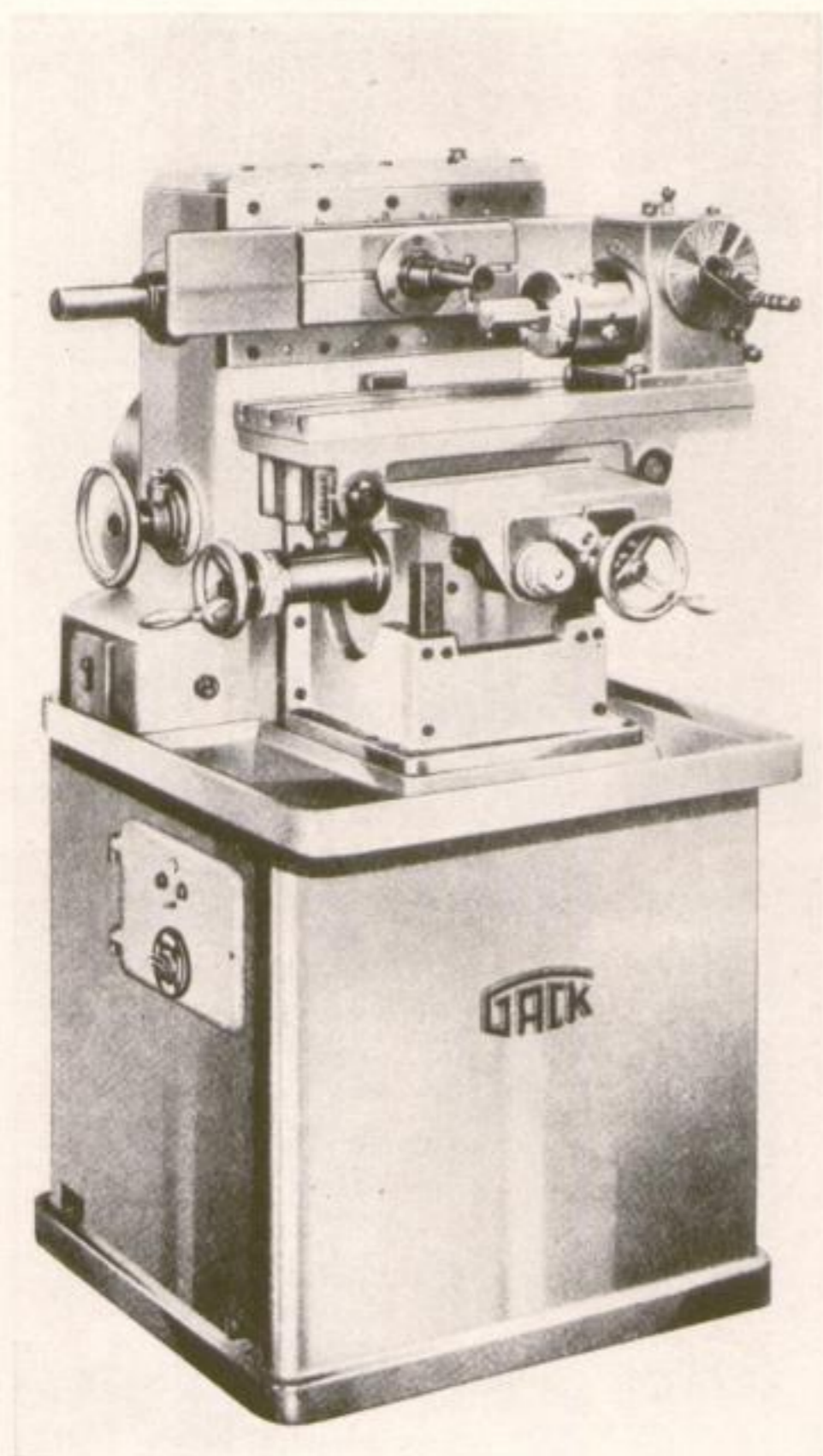
1 Form- und Stempelhobler K 15. Hersteller: Ludwig Gack, Mühlacker/Württemberg
