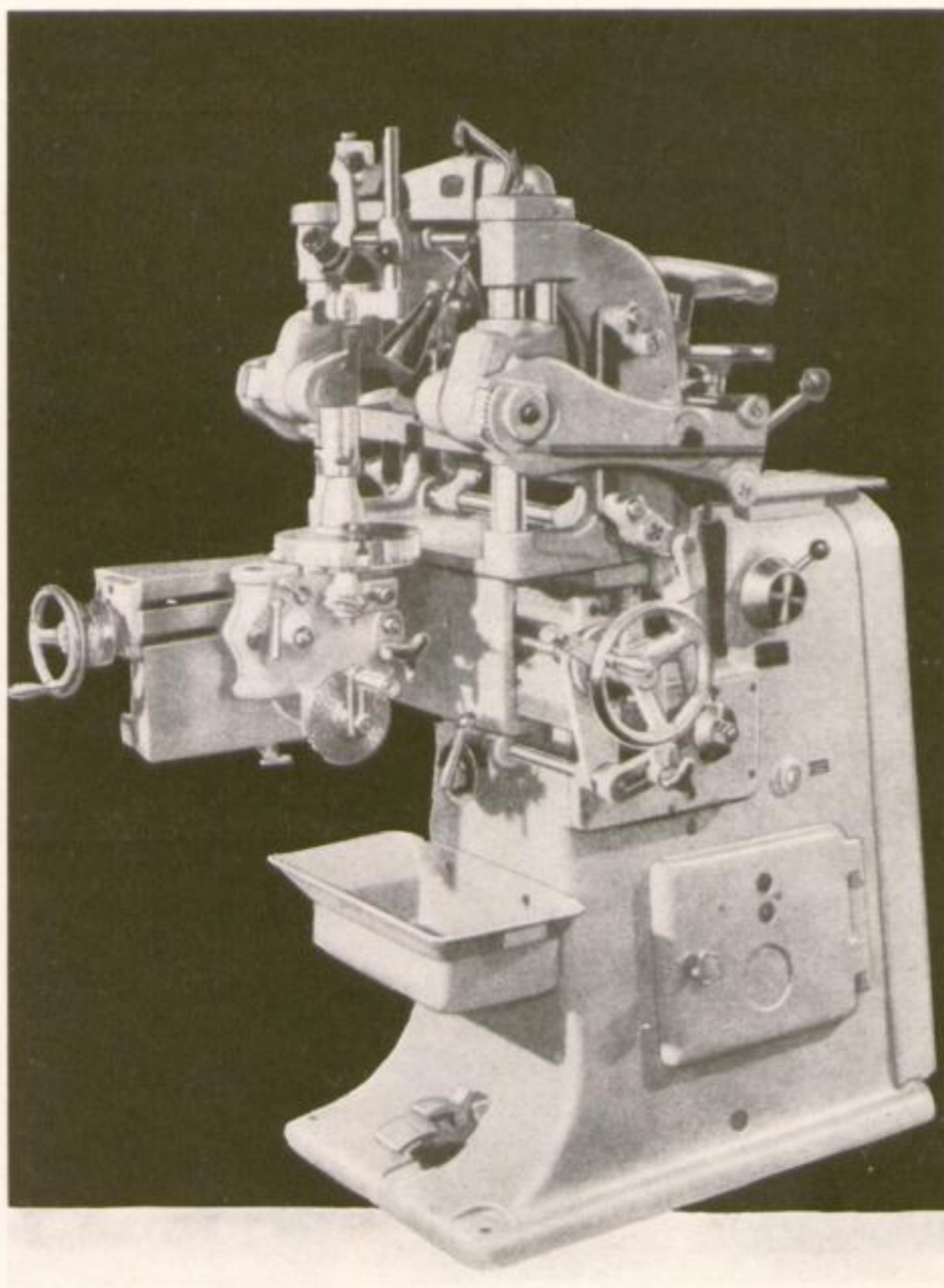
2 Senkrecht-Form- und Stempelstoß- maschine StSF 110, alte Form. Hersteller: VEB UMF Ruhla, Uhren- und Maschinenfabrik, Ruhla
