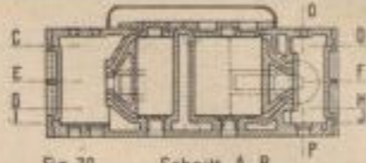
Fig. 70. Schnitt A B.
