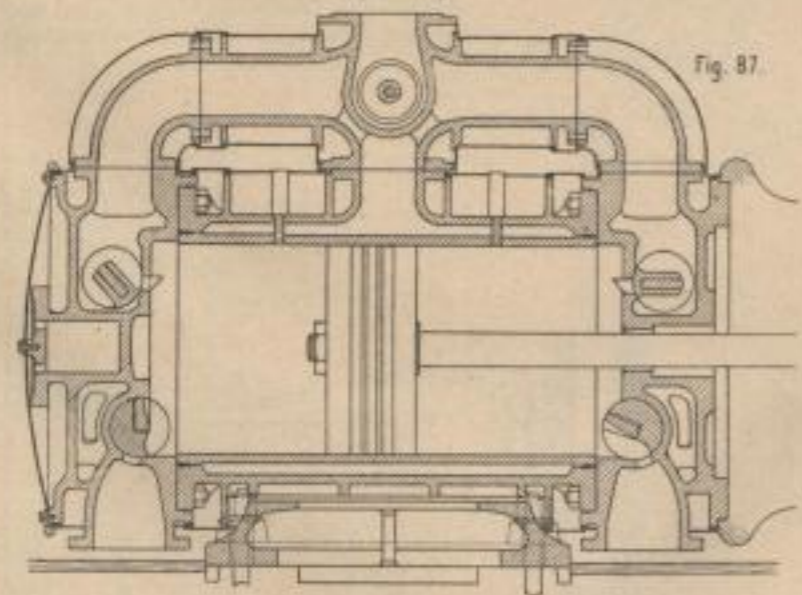
Liegende Maschine von J. Farcot in Saint-Ouen. (83-92)
