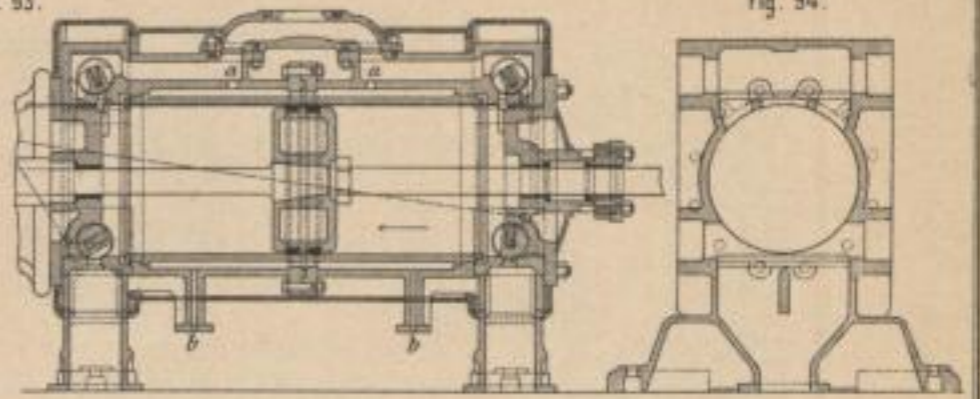
Liegende Maschine von Lecouteux und Garnier in Paris.
