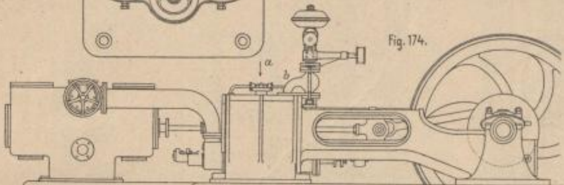
Liegende Maschine von Biatrix und Co. in Saint-Etienne.
