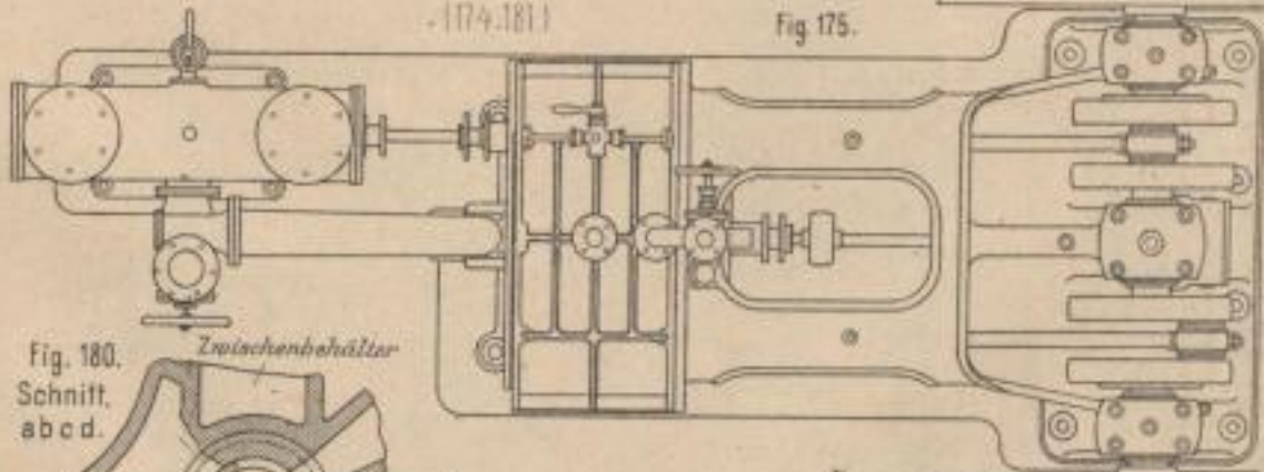
Liegende Maschine von Biatrix und Co. in Saint-Etienne.
