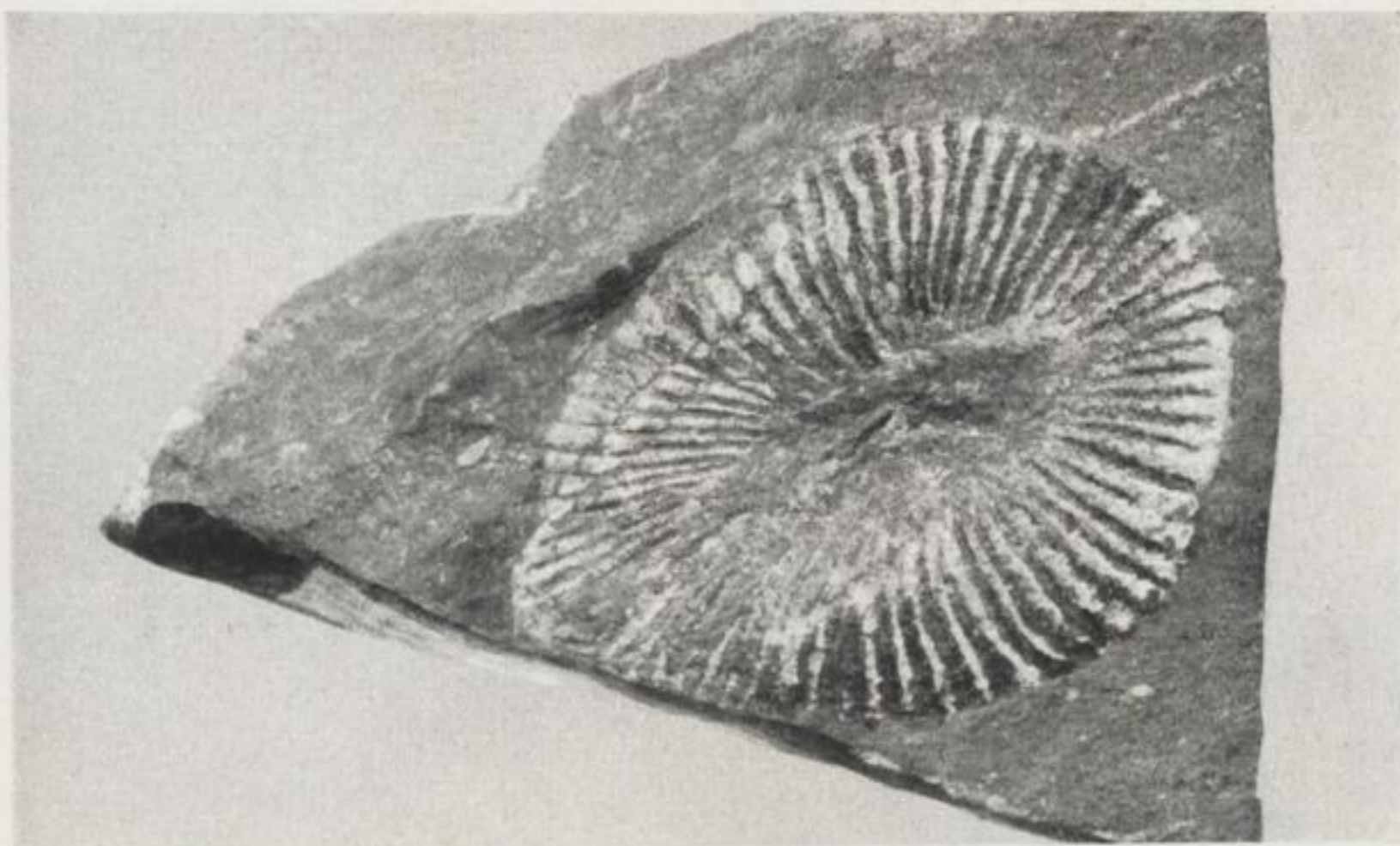
Bild 2. Cyathophyllum helianthoides GOLDF. Obere Manticoceras-Stufe Profil 1 im Bruch am Elsterwehr in Plauen i. V. PL/1 (2fache natürliche Größe)
