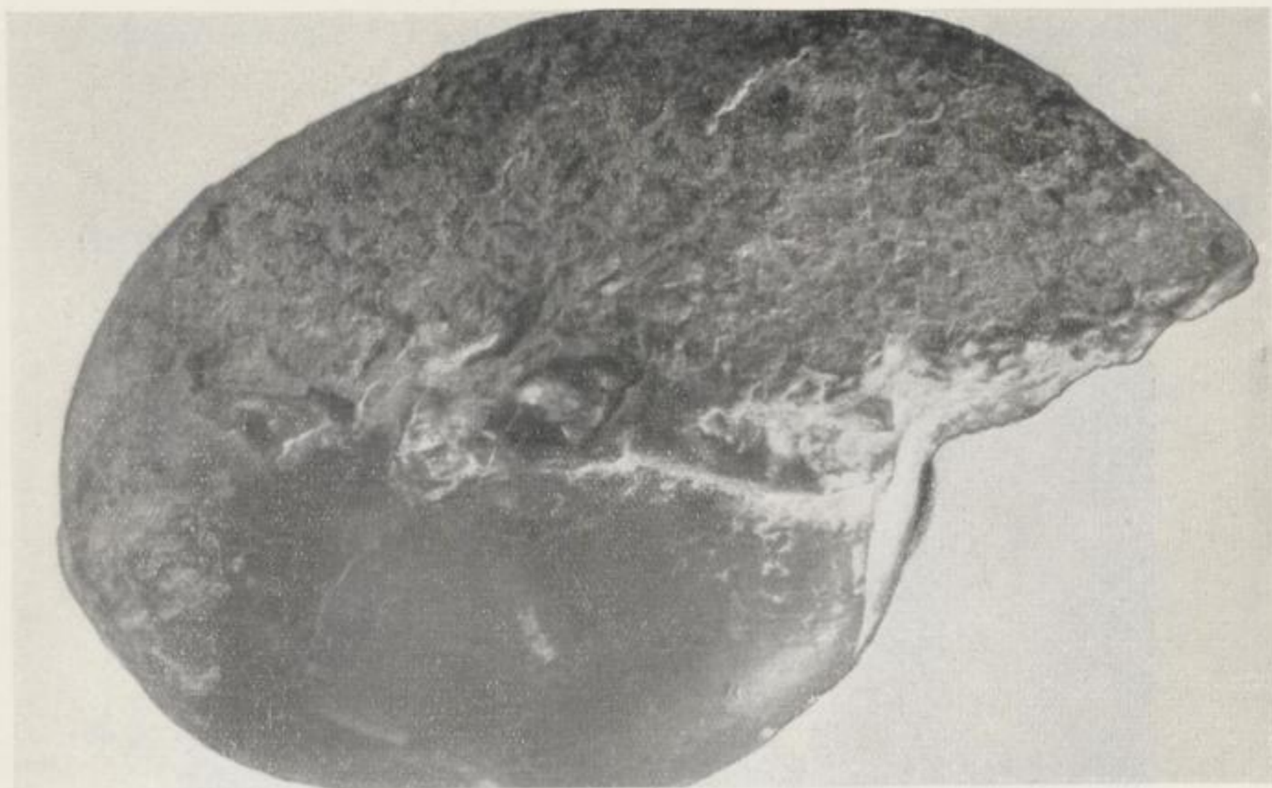
Bild 3. Cyrtoclymenia plicata MSTR. Oberdevon V—VI Ehemaliger Kalkbruch am Kulm bei Oberlosa. 0/1 (2fache natürliche Größe)
