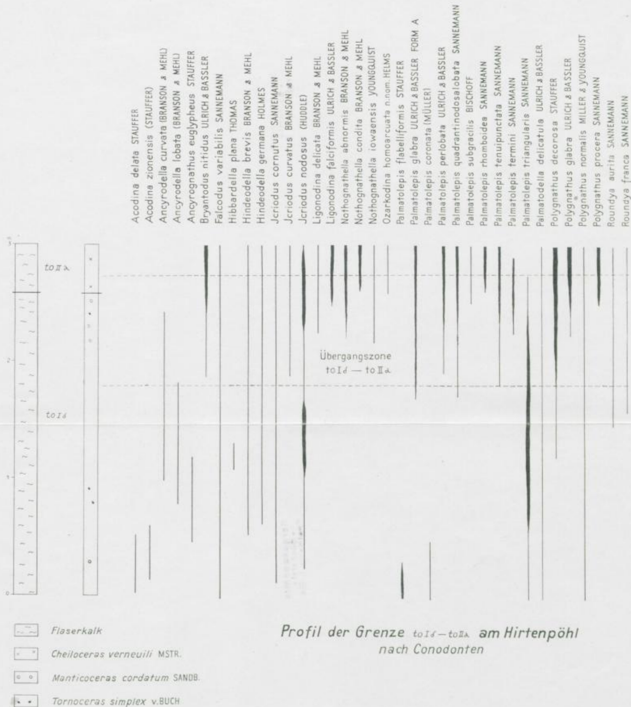
Profil 2 Grenze to Iδ - to IIα am Hirtenpöhl
