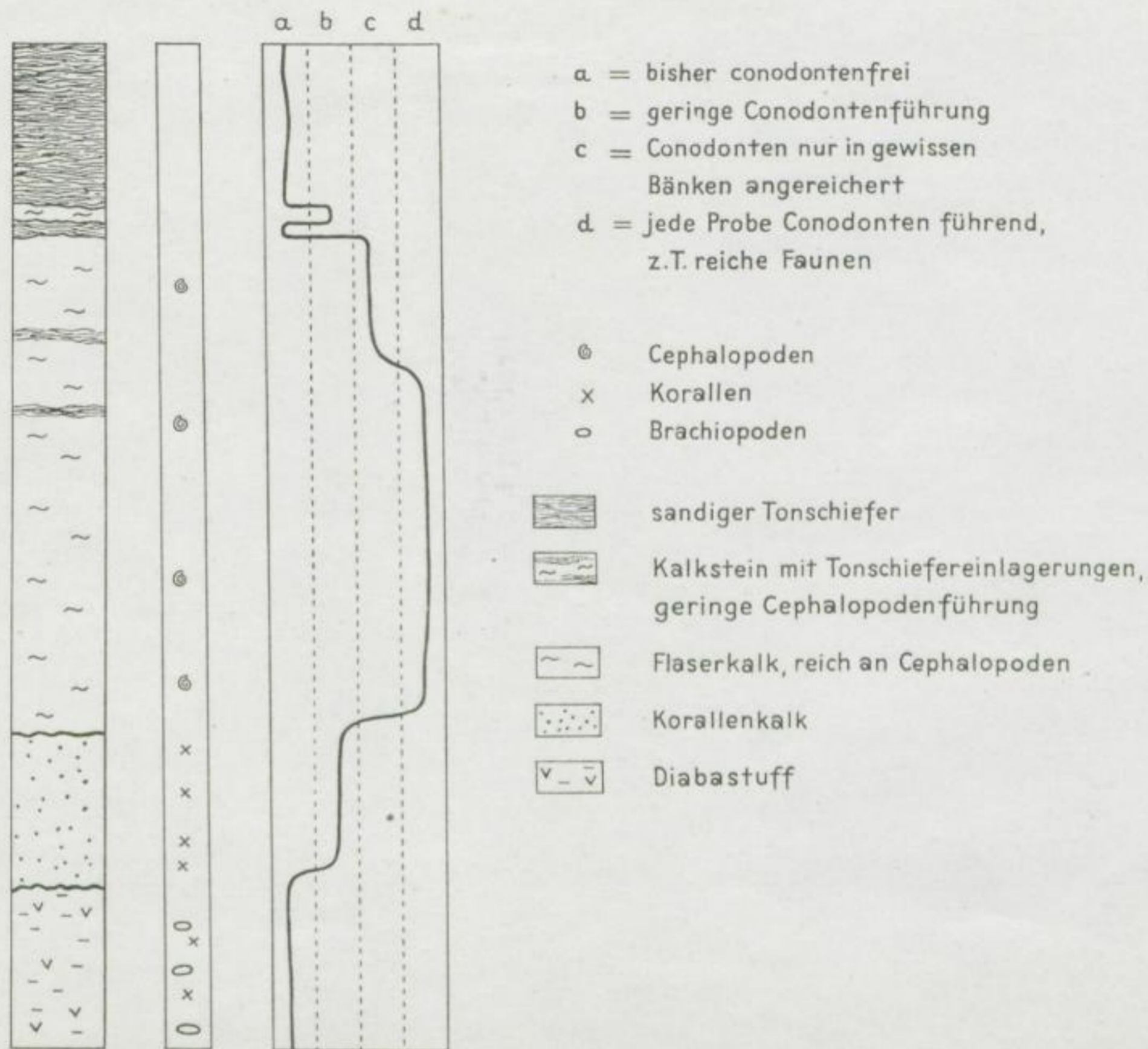
Profil 6 Faziesabhängigkeit und Häufigkeit von Conodontenfaunen im Bereich der Vogtländischen Mulde (schematische Darstellung)
