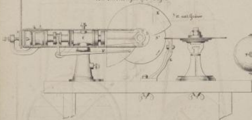
Maschine zum Schneiden der Zähne in Sägeblätter von Ch. Mougin & C. Fig. 3
