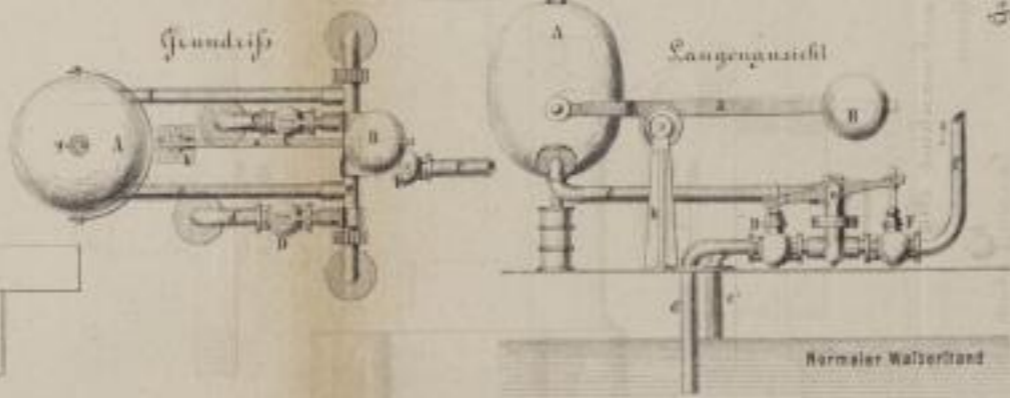
Riedel's selbstthätiger Kesselspeiser Fig. 5 1/2 nat. Größe
