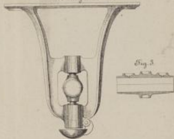
Demier's Anfang-Maschine 1/10 nat. Größe Fig. 3
