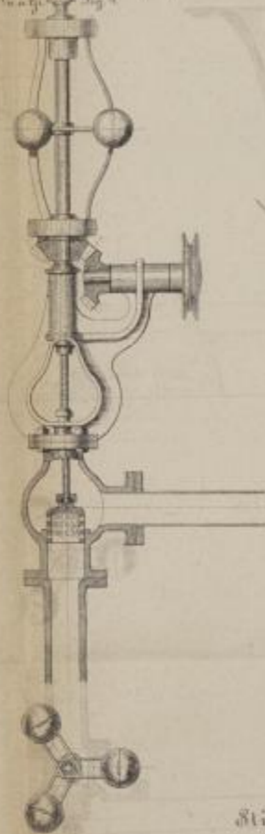
Feder Regulator Lieferung-Louis in New York 1/10 nat. Größe Fig. 4
