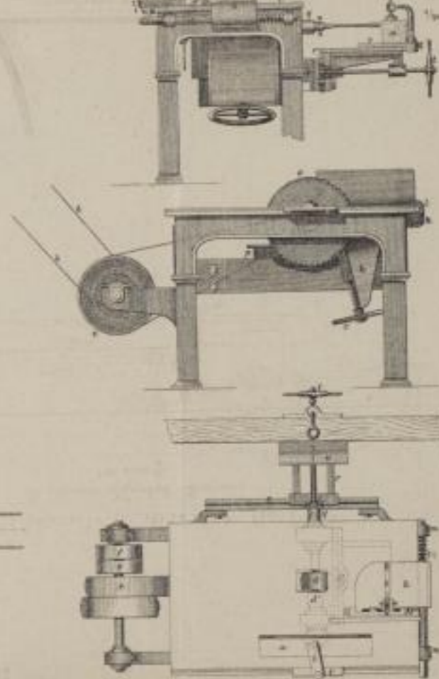
Universal Holz-Bearbeitungs-Maschine Fig. 5 1/10 nat. Größe
