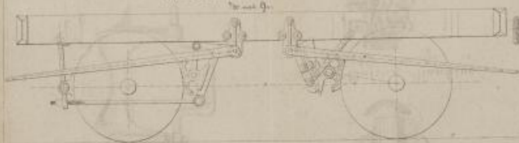
Stilmant'sche Bremse Fig. 6 als Hand Hebel Bremse 1/10 nat. Größe
