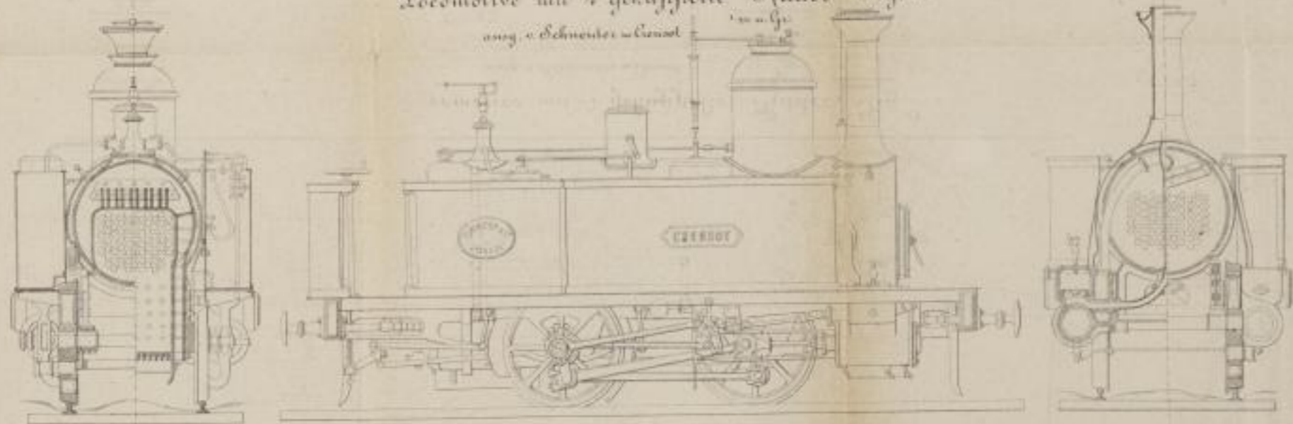
Locomotive mit 4 gekuppelte Räder Fig. 2.
