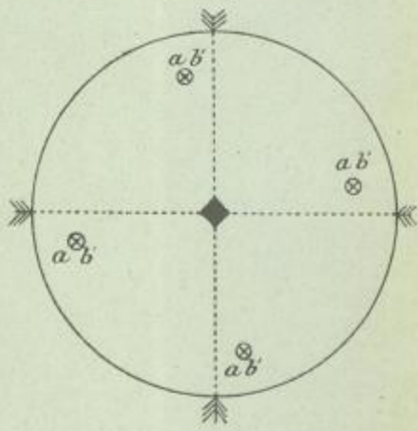
Fig. 36. II. Pyramidale Hemiëdrie. § 16, 4.
