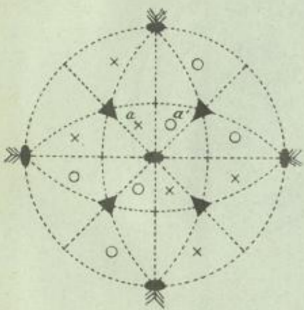
Fig. 29. I. Tetartoëdrie. § 11.
