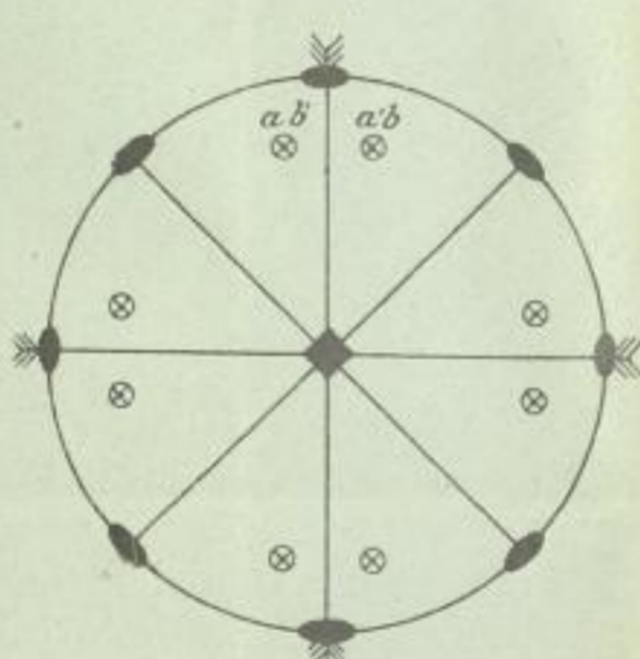
Fig. 33. II. Holoëdrie. § 16, 3.
