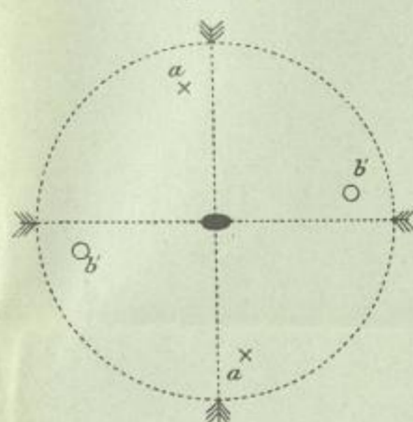
Fig. 34. II. Tetartoëdrie. § 18.
