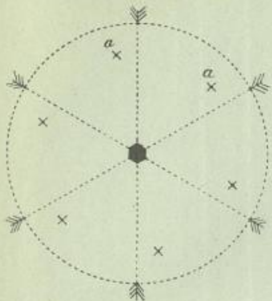
Fig. 50. III. Hemimorphie der trapezoëdr. und pyramid. Hemiëdrie. § 12.
