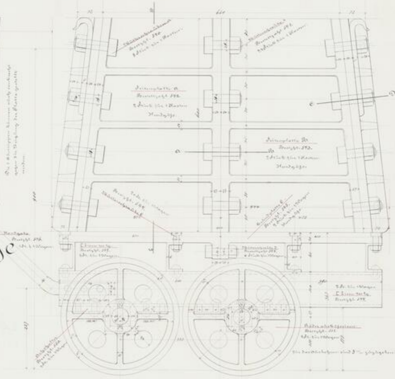
Fig. 1. Hängen - Ansicht.
