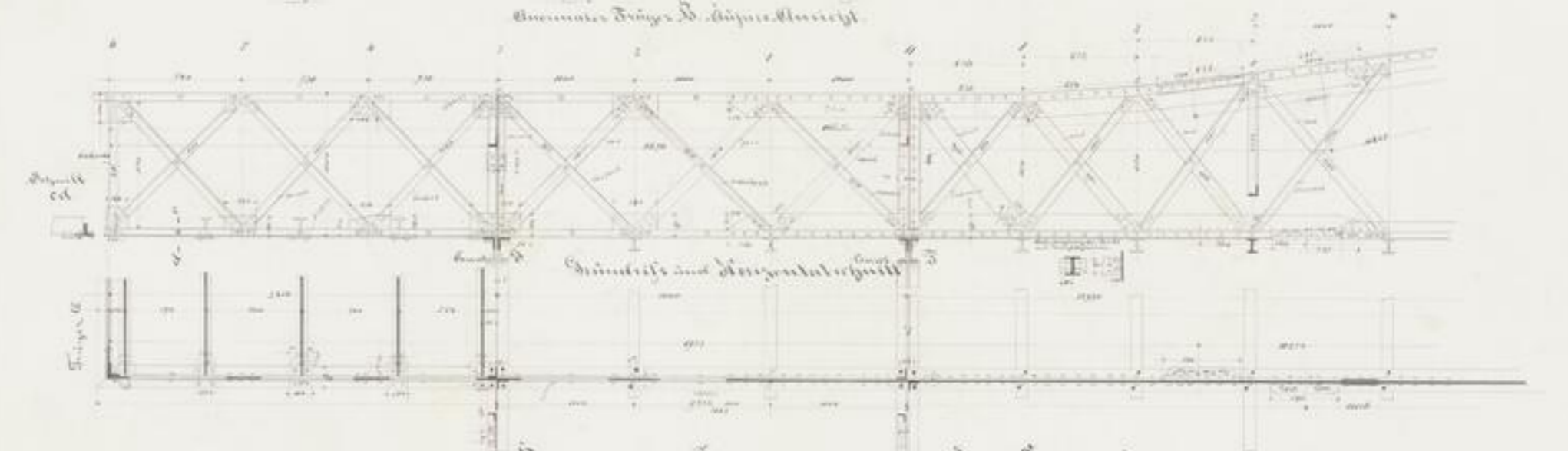
Die normalen Druckträger A und B der Erzbrücke.
