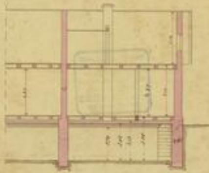
Längenschnitt.
