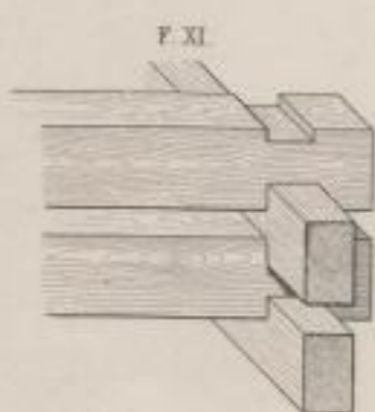
Details von Eckverbänden bei Schweizer Blockhäusern
