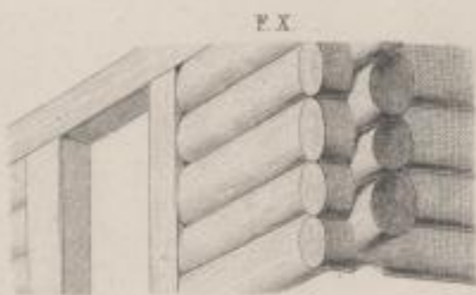
Details von Eckverbänden bei Schweizer Blockhäusern
