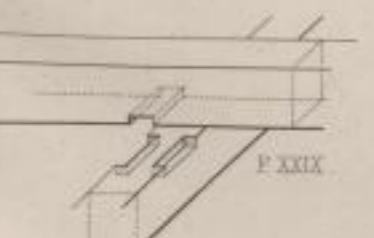
Doppelkamm.
