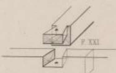
Schwalbenschwanzförmiges Blatt.
