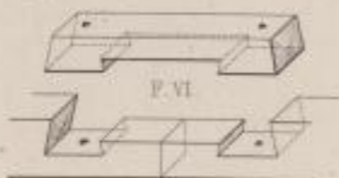
Stoß mit eingesetztem schräg geschnittenem Haken.
