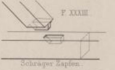
Gerader Zapfen.
