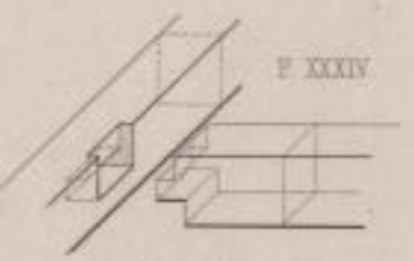
Geächter Zapfen.
