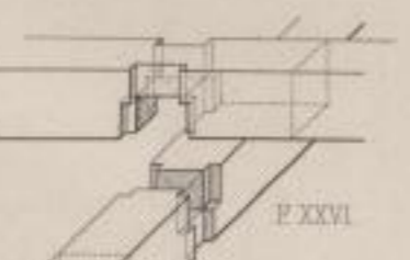
Schwalbenschwanzförmiges Blatt (einerseitig geschlitten).
