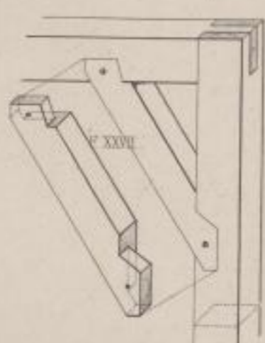
Angeblatteten Winkelband.
