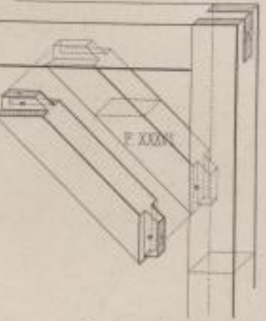
Jagdzapfen.
