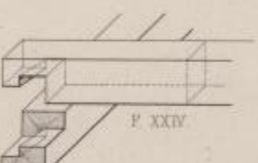
Schräges Hakenblatt (Rekverbindung).
