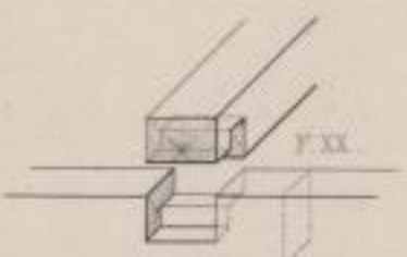
Hakenblatt.
