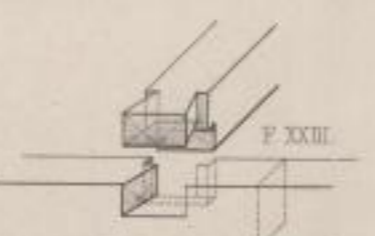
Schwalbenschwanzförmiges Blatt mit Brüstung.
