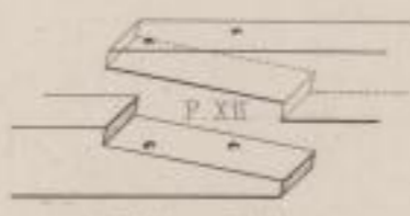
Schräges Blatt.
