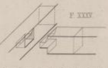
Brustzapfen mit geradem u. schrägen Schnitt.
