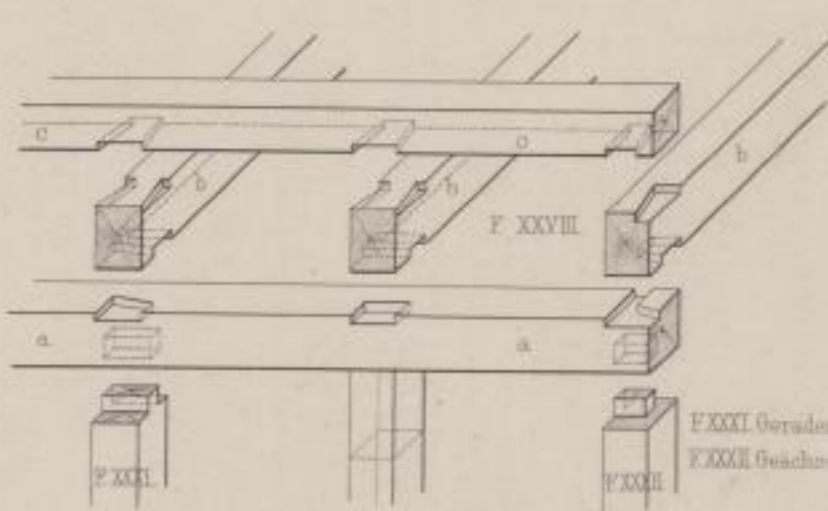
Verkammungen zwischen Rahmholz, Balken u. Saumschwelle beim Fachwerksbau.
