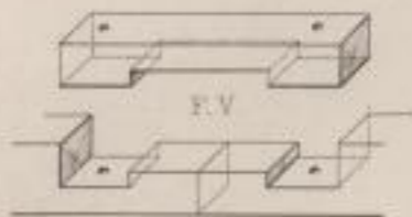
Stoß mit eingesetztem geradem Haken.
