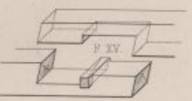
Gerades Hakenblatt mit schrägen Schnitten u. Keil.
