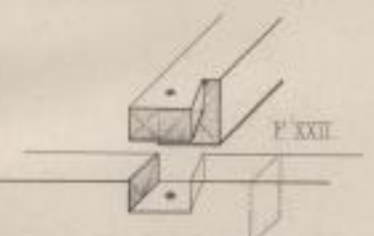
Schwalbenschwanzförmiges Blatt (einerseitig geschlitten).
