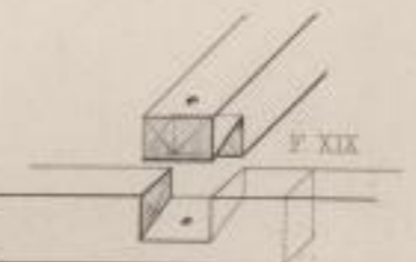
Schräges Blatt.
