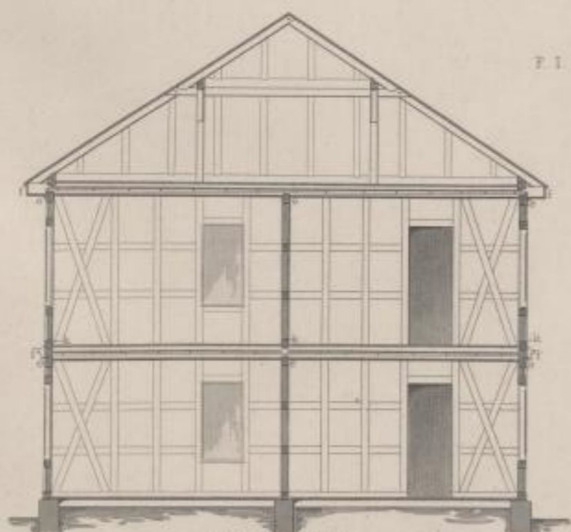
F I q Querschnitt nach r-a
