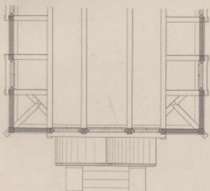
F II g Grundriss
