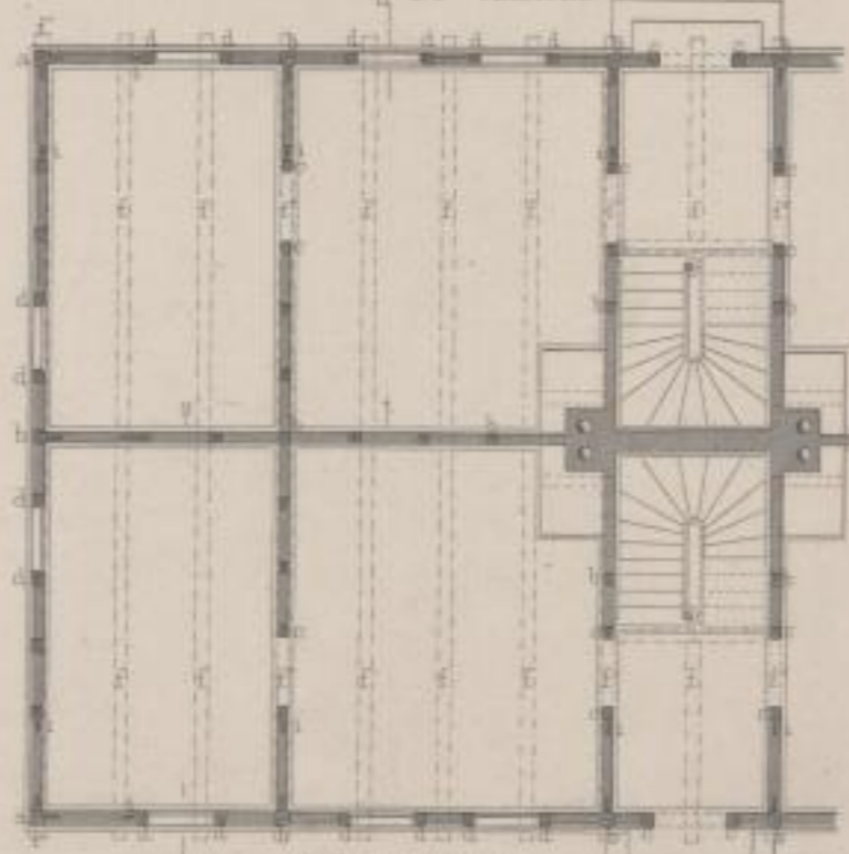
F I g Grundriss
