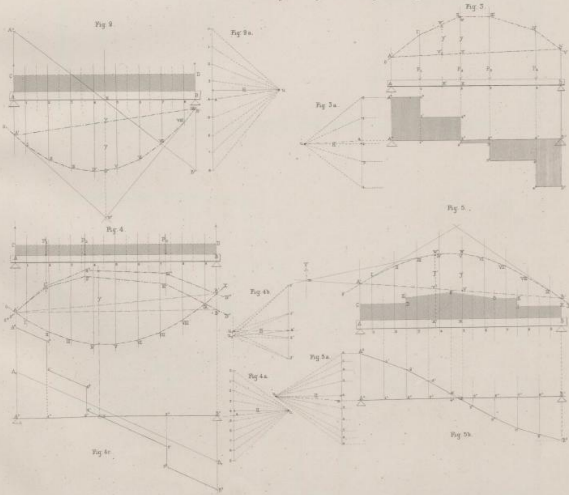
Graphische Bestimmung der Maximalmomente für frei auf zwei Stützen aufliegende Träger und beliebige Belastungen.
