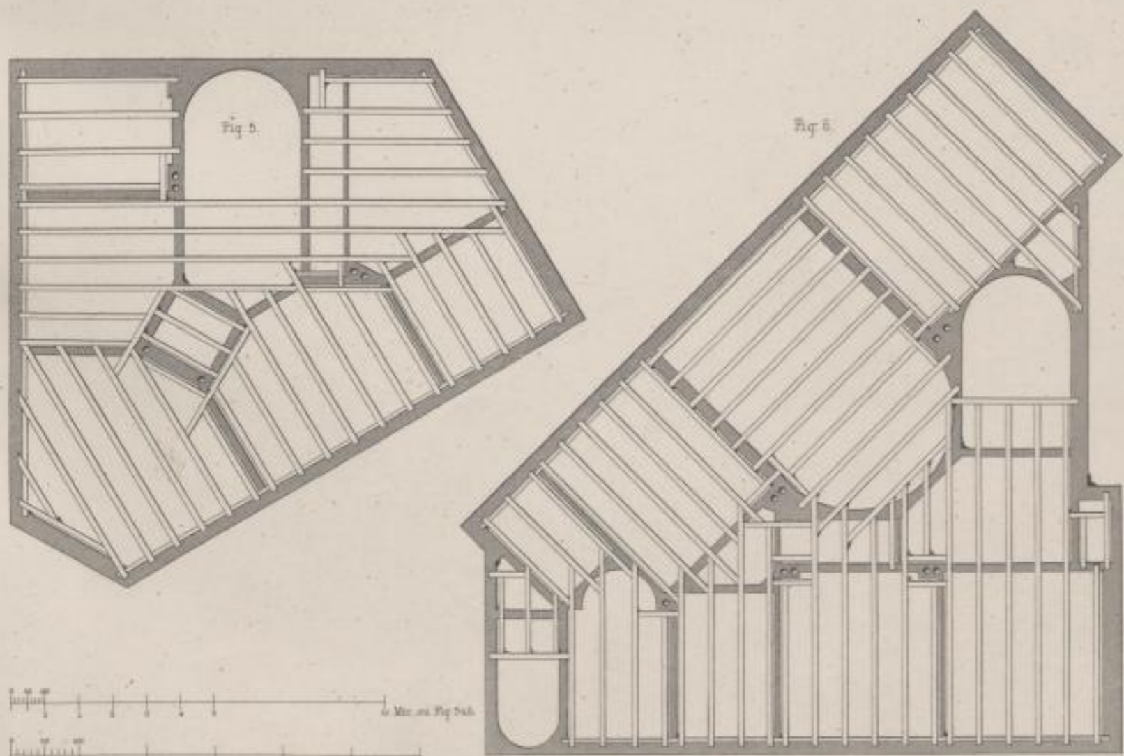
Balkenlagen über irreguläre Räume.
