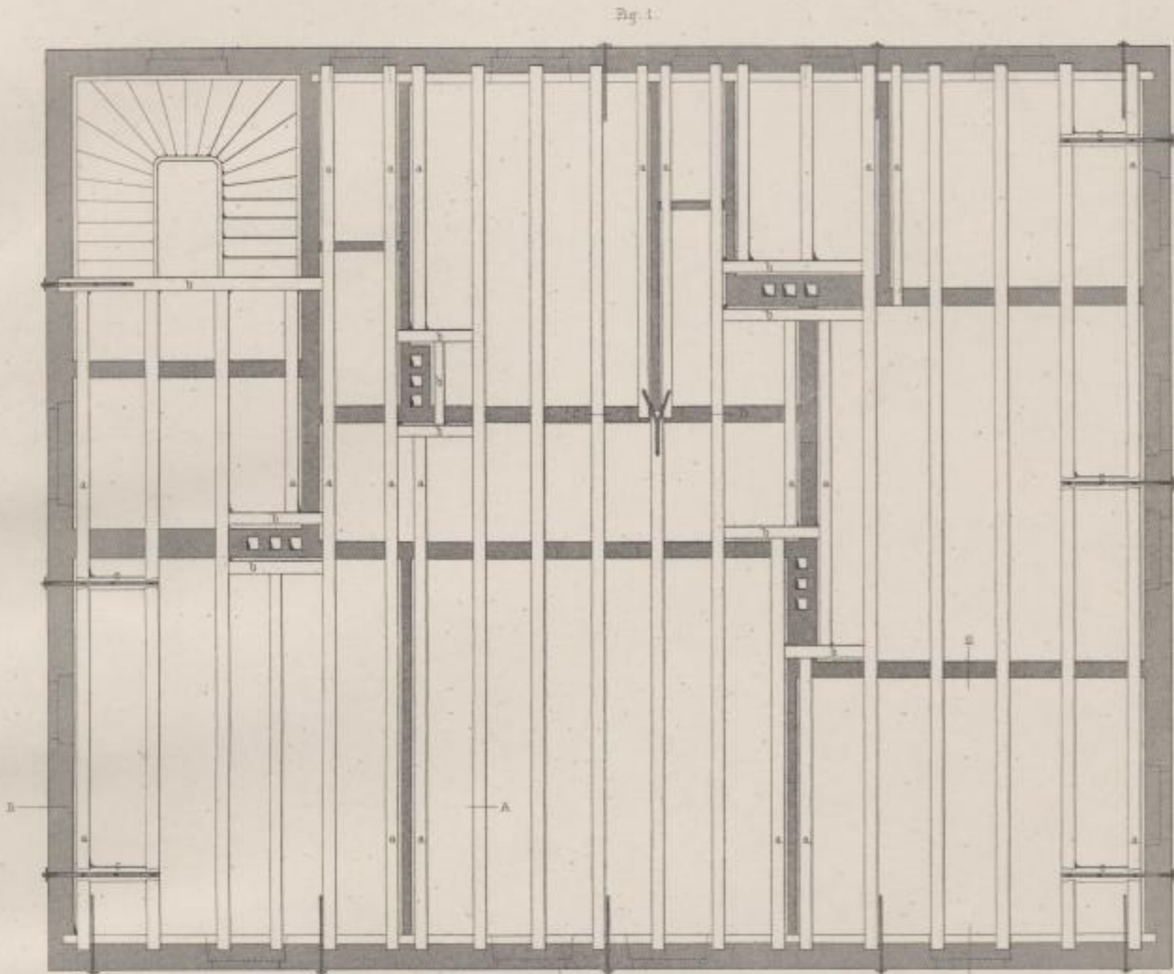
Balkenlage über regulär-rechteckigen Raum.
