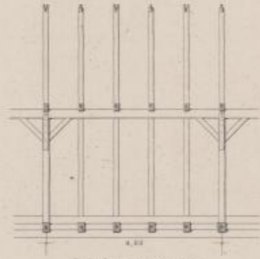
F.II. Längenschnitt.
