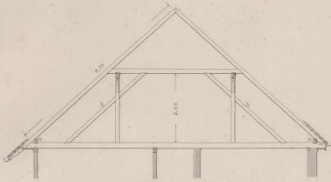
F.I. Querschnitt.
