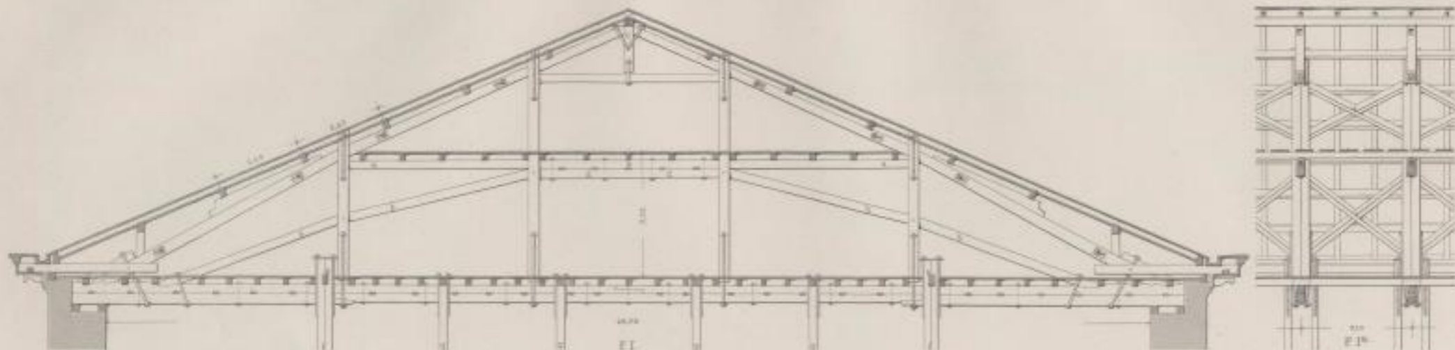
Dachstuhl, dem Hoftheater in München angehörend
