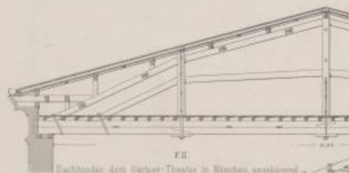
Dachstuhl dem Gärtner-Theater in München angehörend
