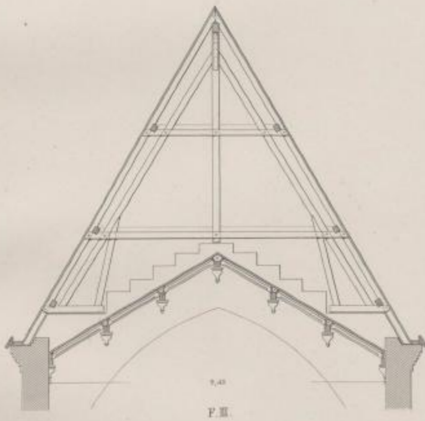
Dachstuhl der Brigittenauer-Kirche bei Wien. (nach Fr. Schmidt)
