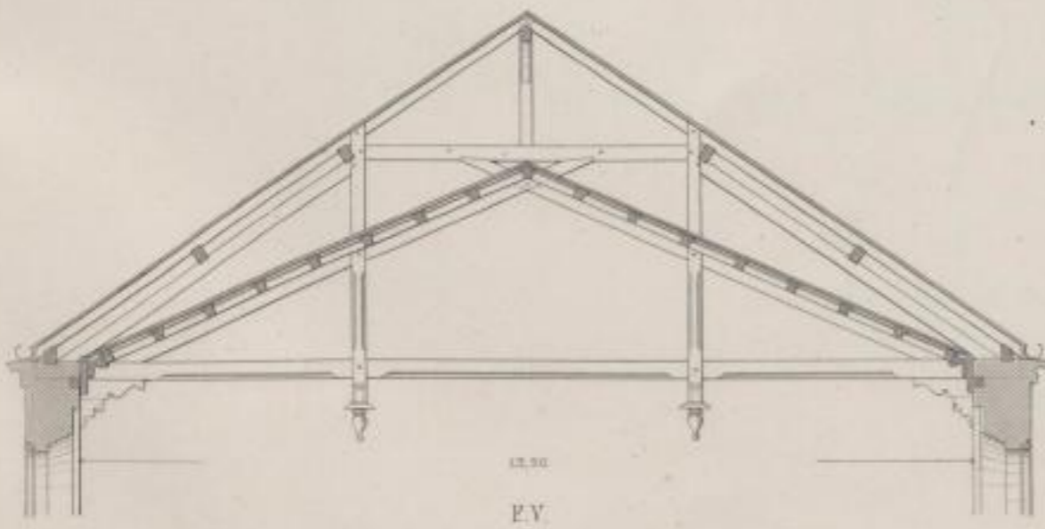
Kirchendachstuhl nach Stüler.
